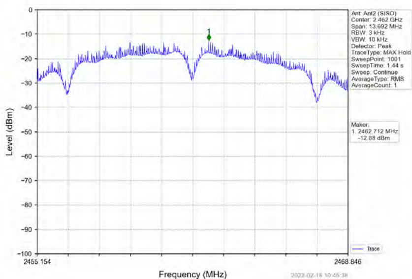
802.11b_HCH_2462MHz_Ant2 (SISO)_NTNV
