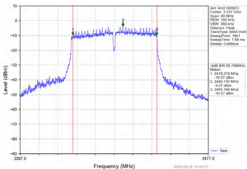
802.11n(HT40) MCH_2437MHz_Ant2 (MIMO) NTVN
