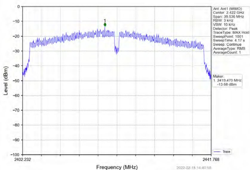
802.11n(HT40)_LCH_2422MHz_Ant1 (MIMO)_NTNV
