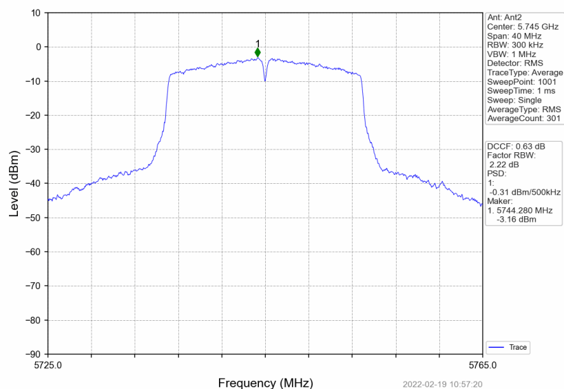
802.11n(HT20) LCH_5745MHz_MIMO_NTNV
