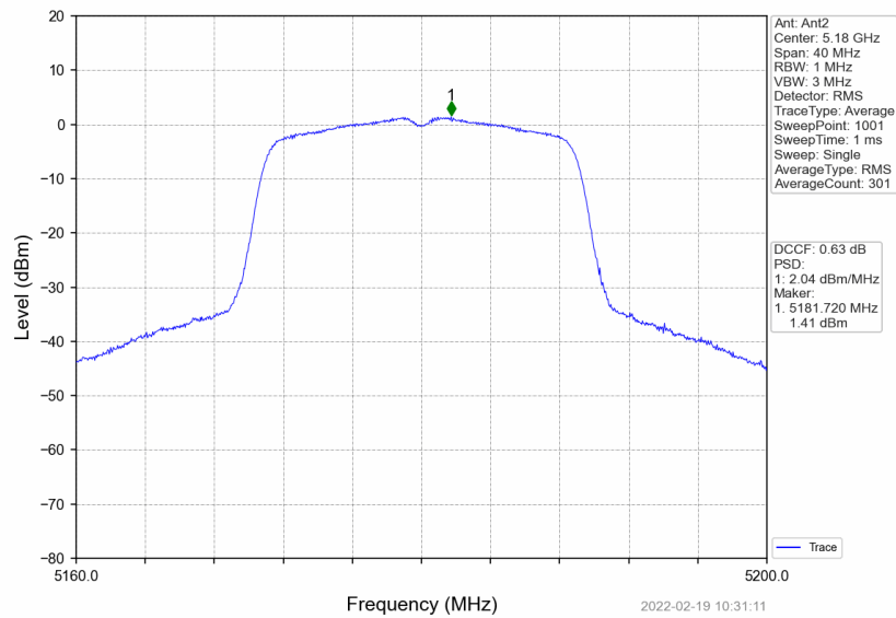
802.11n(HT20)_LCH_5180MHz_MIMO_NTNV
