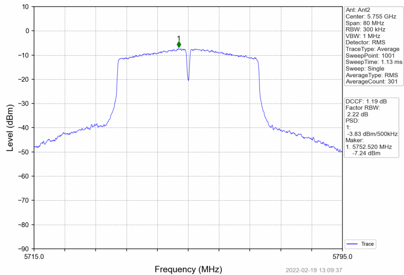
802.11n(HT40)_LCH_5755MHz_MIMO_NTNV
