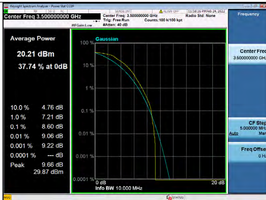
Band42H_10MHz_QPSK_MCH_3500MHz_RB_50_0_NTNV
