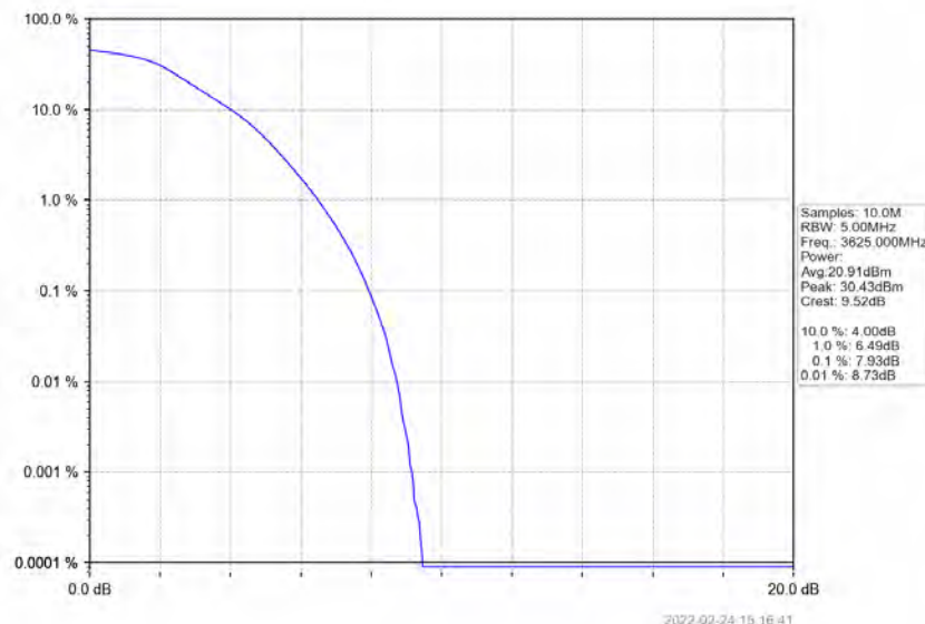
Band48_5MHz_QPSK_MCH_3625MHz_RB_25_0_NTNV
