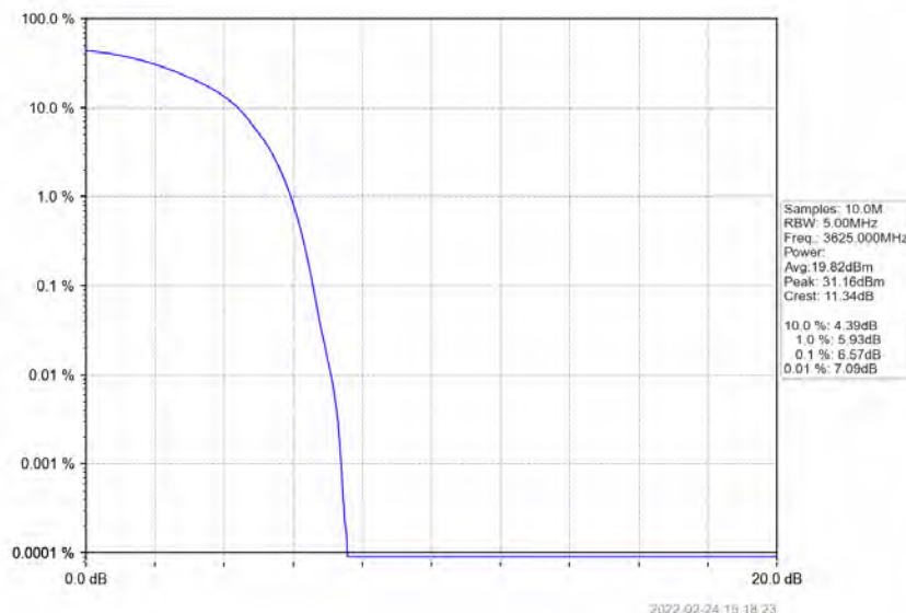
Band48_10MHz_QPSK_MCH_3625MHz_RB_50_0_NTNV
