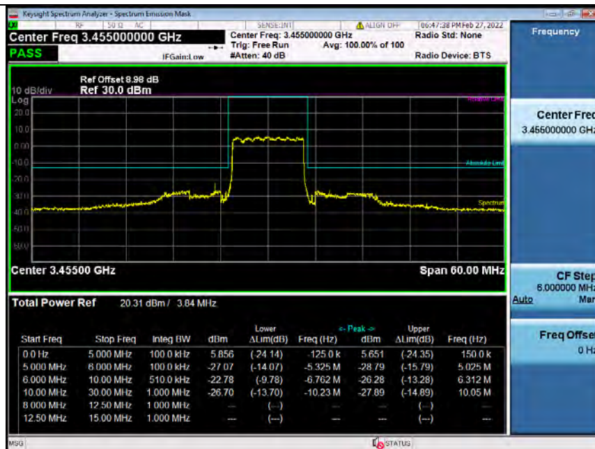
Band42H_10MHz_QPSK_LCH_3455MHz_RB_50_0_NTNV_Bandedge
