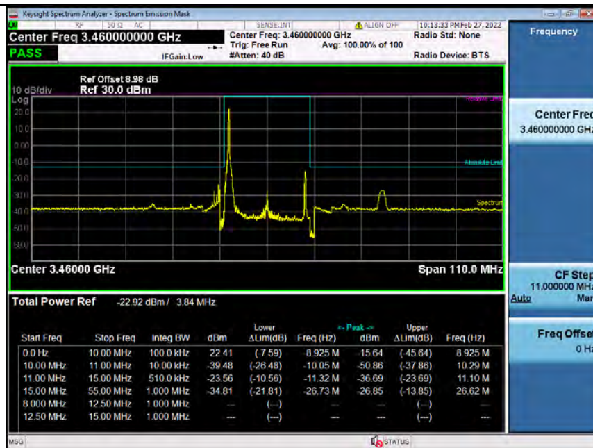
Band42H_20MHz_QPSK_LCH_3460MHz_RB_100_0_NTNV_Bandedge
