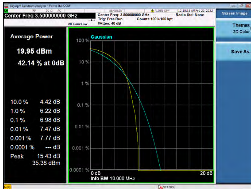
Band42H_20MHz_QPSK_MCH_3500MHz_RB_100_0_NTNV
