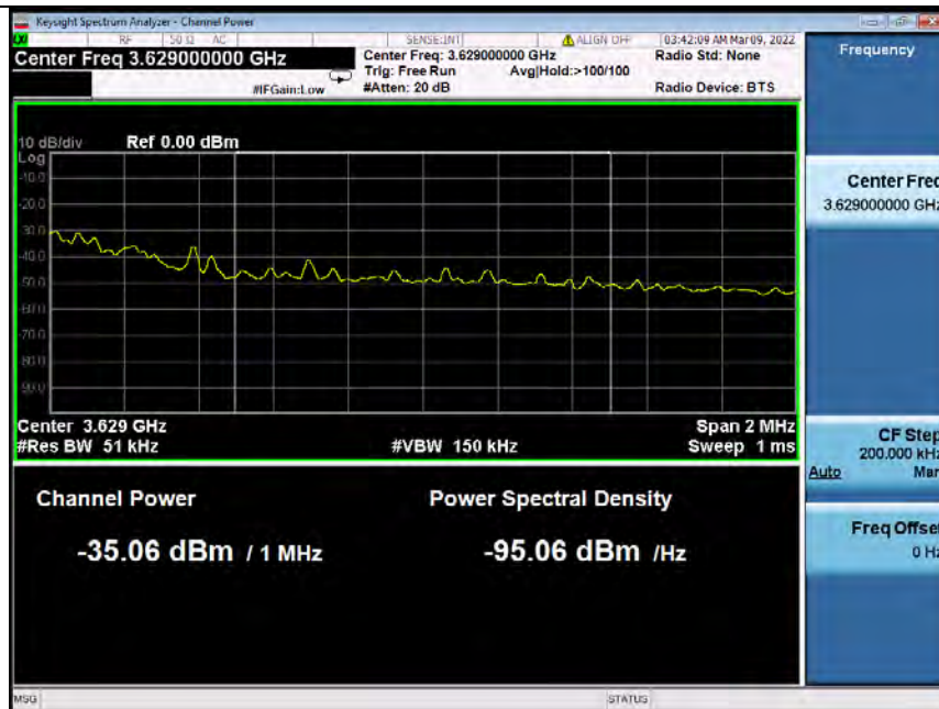
Band48_5MHz_QPSK_MCH_3625MHz_RB_25_0_NTNV
