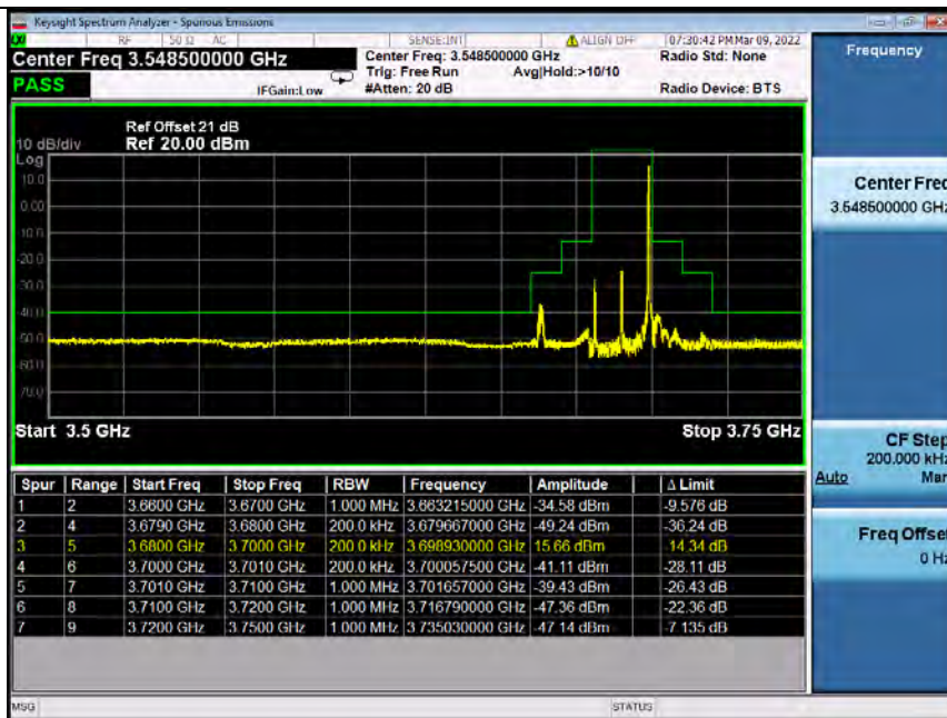
Band48_20MHz_16QAM_HCH_3690MHz_RB_100_0_NTNV
