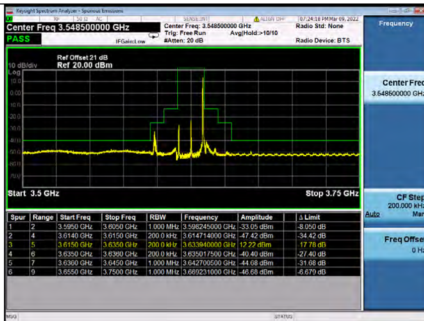
Band48_20MHz_16QAM MCH_3625MHz_RB_100_0_NTNV
