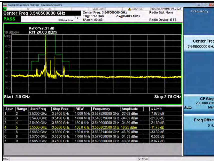
Band48_15MHz_QPSK_LCH_3557.5MHz_RB_1_74_NTNV
