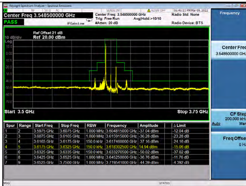
Band48_15MHz_64QAM_MCH_3625MHz_RB_1_74_NTNV
