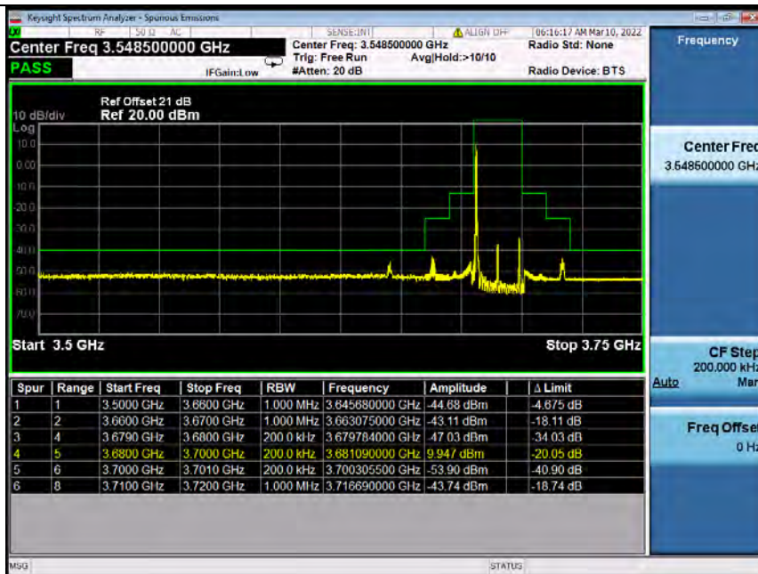
Band48_20MHz_QPSK_HCH_3690MHz_RB_1_99_NTNV
