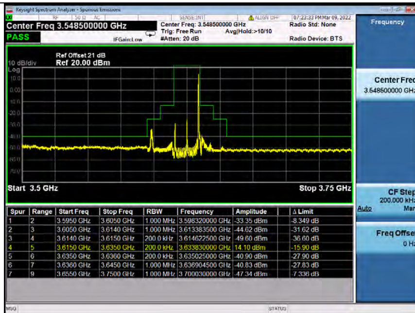
Band48_20MHz_QPSK_MCH_3625MHz_RB_100_0_NTNV
