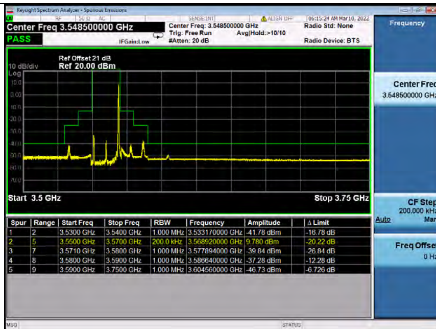
Band48_20MHz_QPSK_LCH_3560MHz_RB_1_99_NTNV
