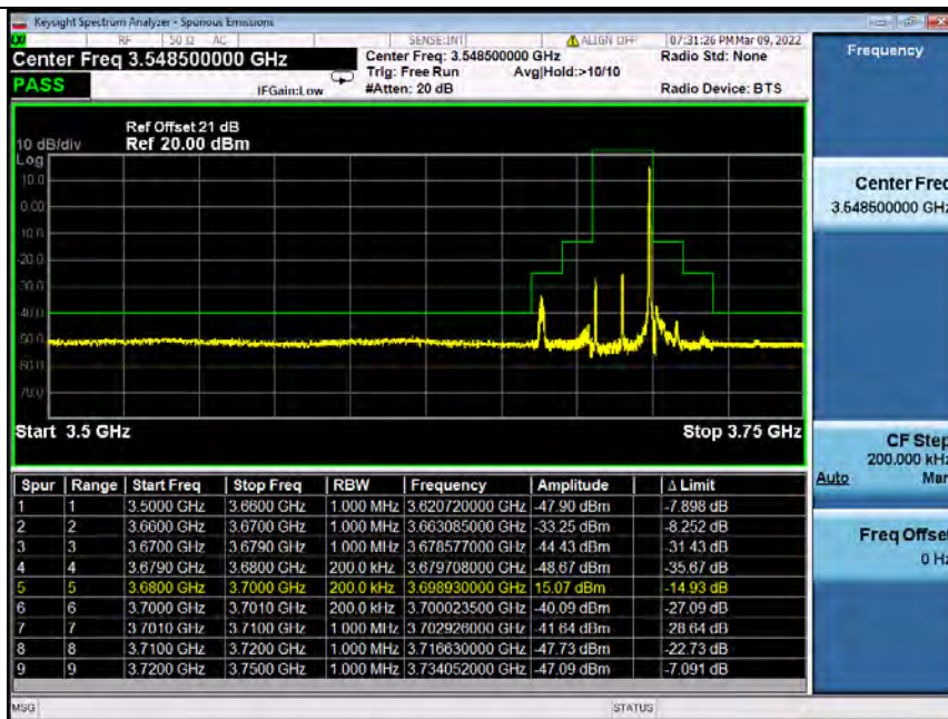
Band48_20MHz_QPSK_HCH_3690MHz_RB_100_0_NTNV
