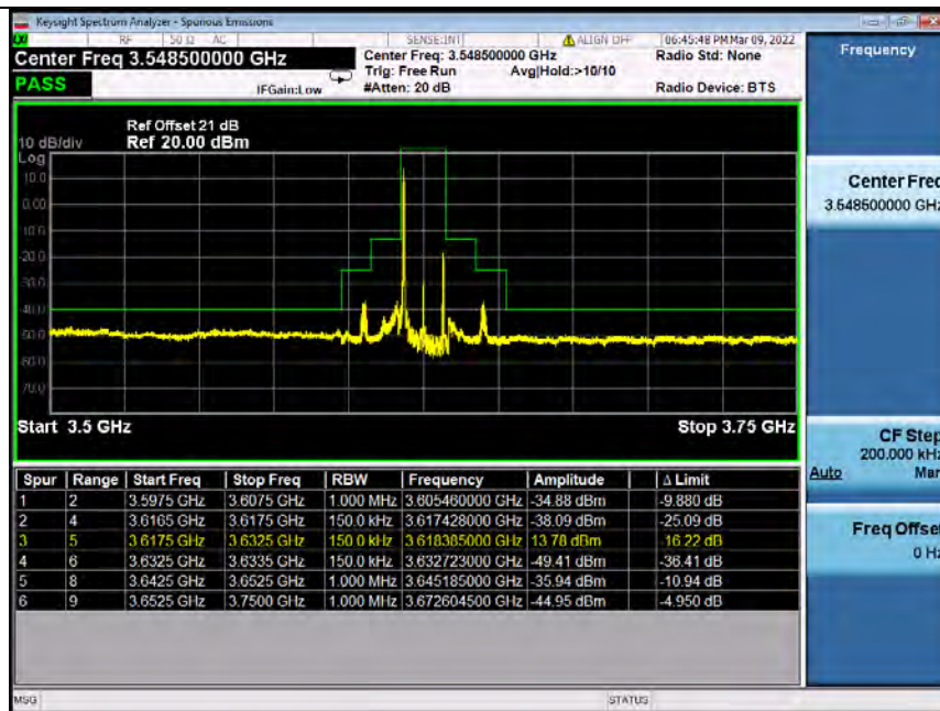
Band48_15MHz_16QAM_MCH_3625MHz_RB_1_74_NTNV
