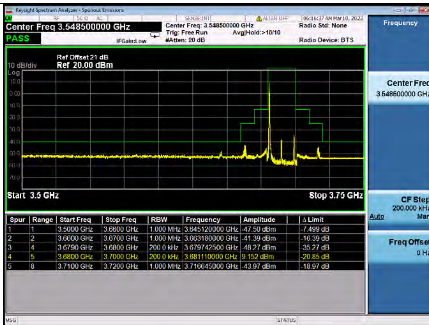
Band48_20MHz_16QAM_HCH_3690MHz_RB_1_99_NTNV
