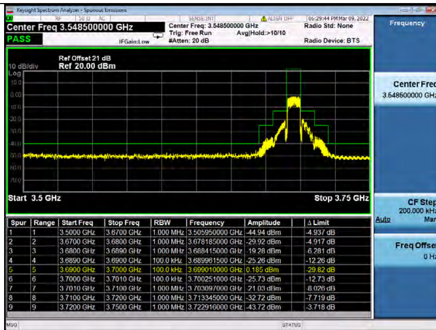
Band48_10MHz_QPSK_HCH_3695MHz_RB_50_0_NTNV
