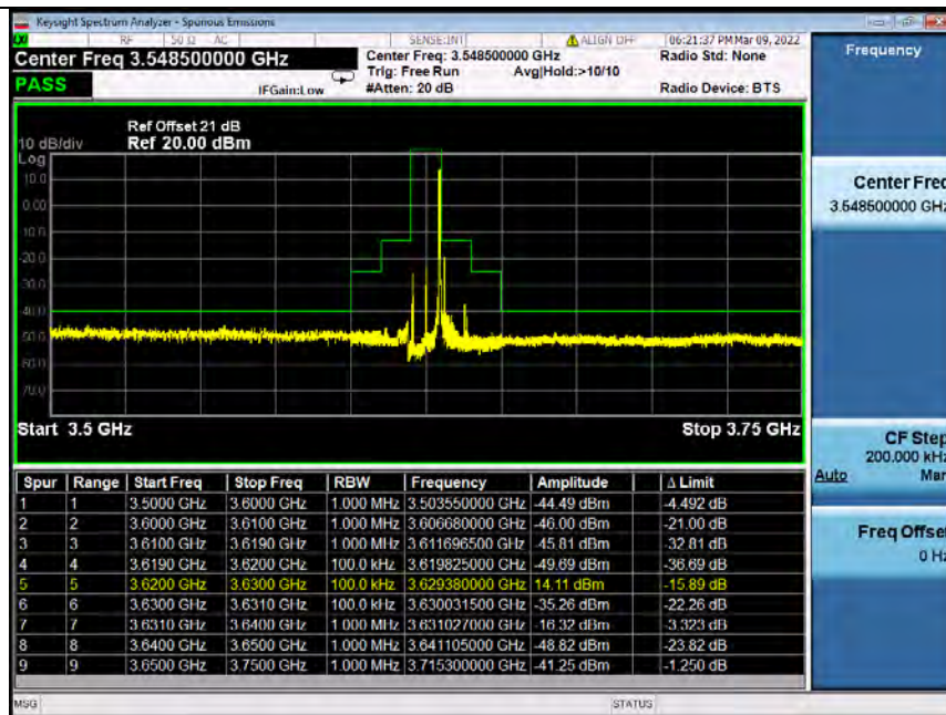
Band48_10MHz_QPSK_MCH_3625MHz_RB_50_0_NTNV
