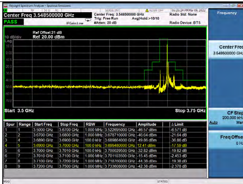
Band48_10MHz_QPSK_HCH_3695MHz_RB_50_0_NTNV
