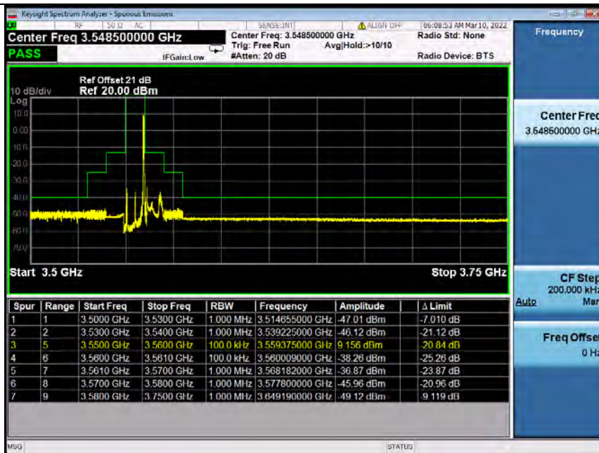
Band48_10MHz_16QAM_LCH_3555MHz_RB_50_0_NTNV
