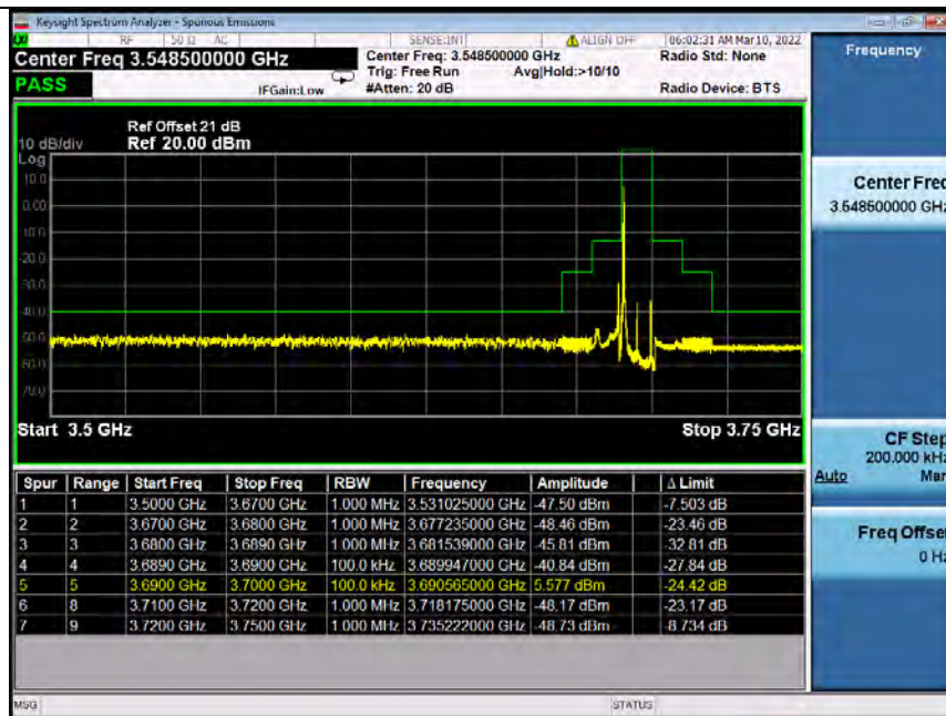
Band48_10MHz_QPSK_HCH_3695MHz_RB_1_49_NTNV
