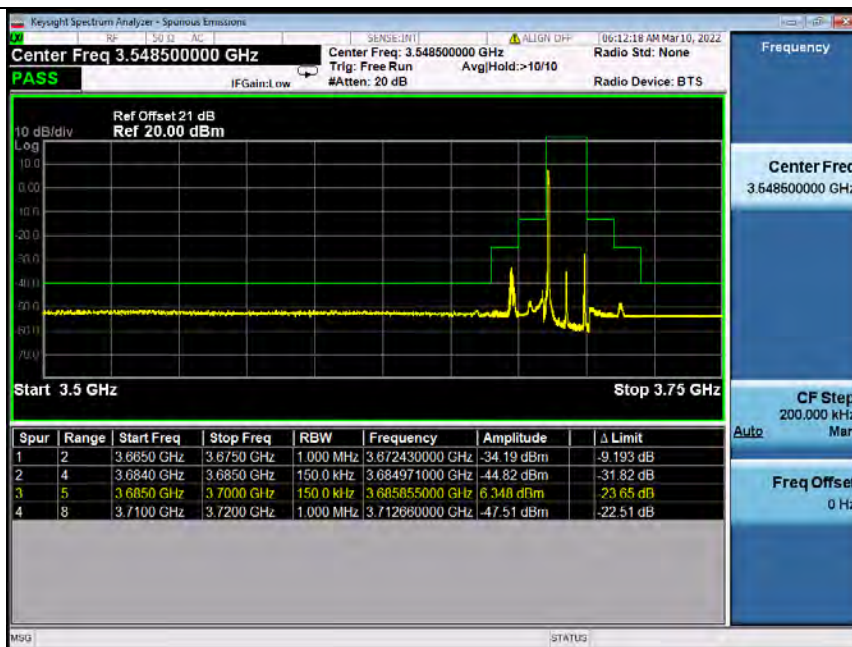
Band48_15MHz_16QAM_HCH_3692.5MHz_RB_1_74_NTNV
