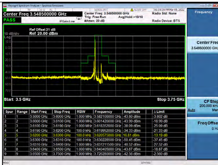
Band48_10MHz_64QAM_MCH_3625MHz_RB_1_49_NTNV
