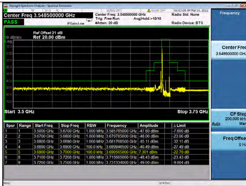
Band48_10MHz_16QAM_HCH_3695MHz_RB_1_49_NTNV
