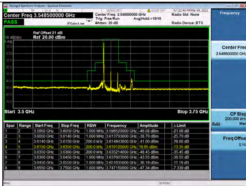
Band48_20MHz_64QAM_MCH_3625MHz_RB_1_99_NTNV
