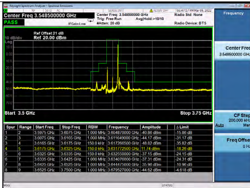
Band48_15MHz_QPSK_MCH_3625MHz_RB_75_0_NTNV
