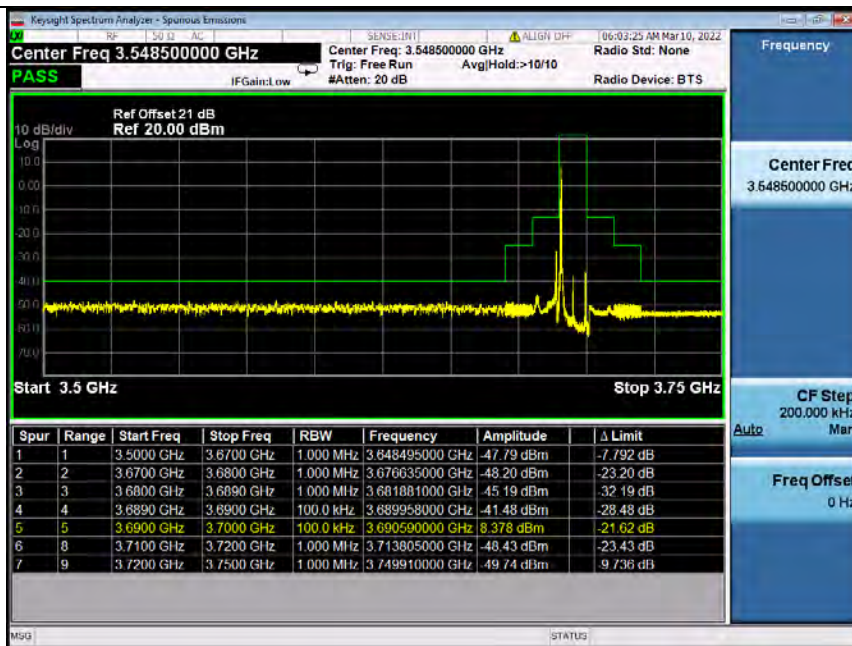
Band48_10MHz_64QAM_HCH_3695MHz_RB_1_49_NTNV
