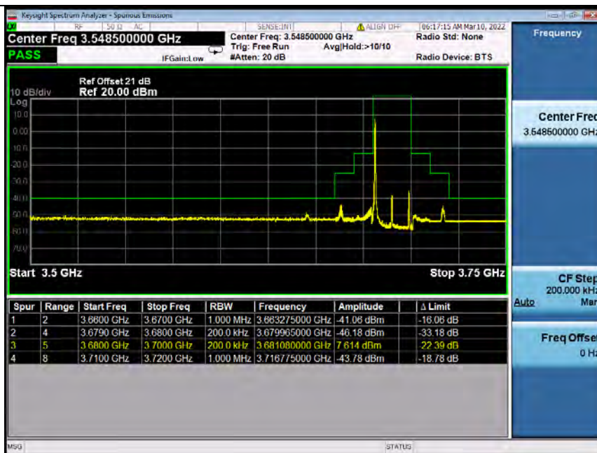
Band48_20MHz_64QAM_HCH_3690MHz_RB_1_99_NTNV
