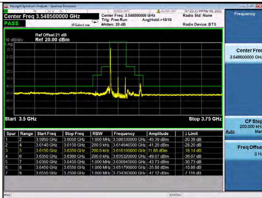
Band48_20MHz_16QAM_MCH_3625MHz_RB_1_99_NTNV
