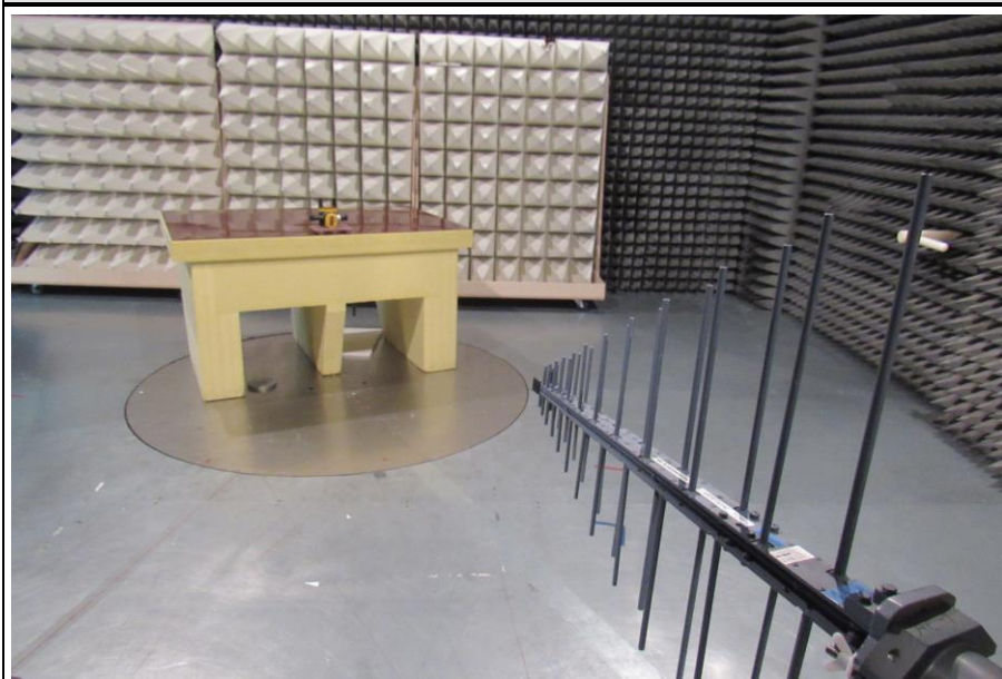
TEST SETUP HL 223
