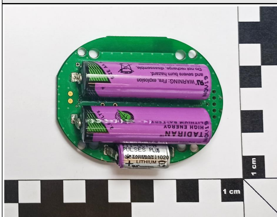
EUT PCB BOTTOM SIDE
