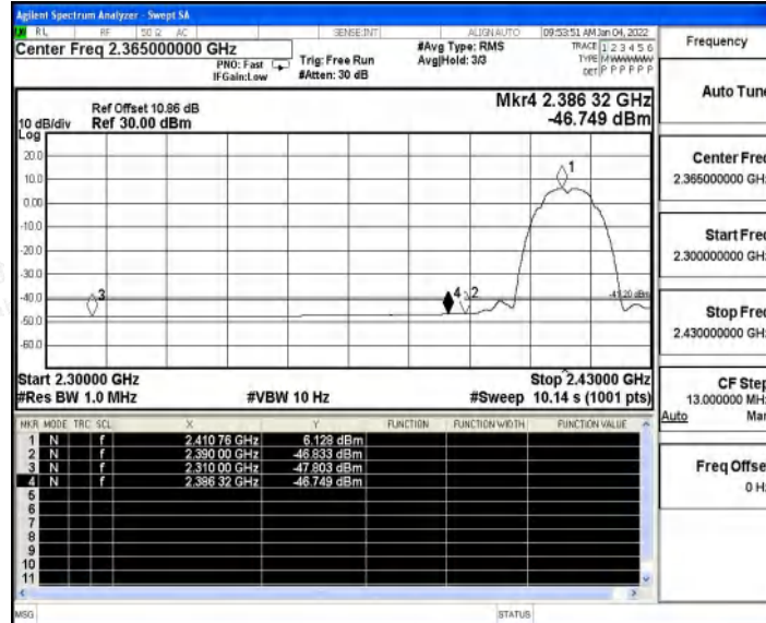
11B_Ant0_Low_2412_Peak
