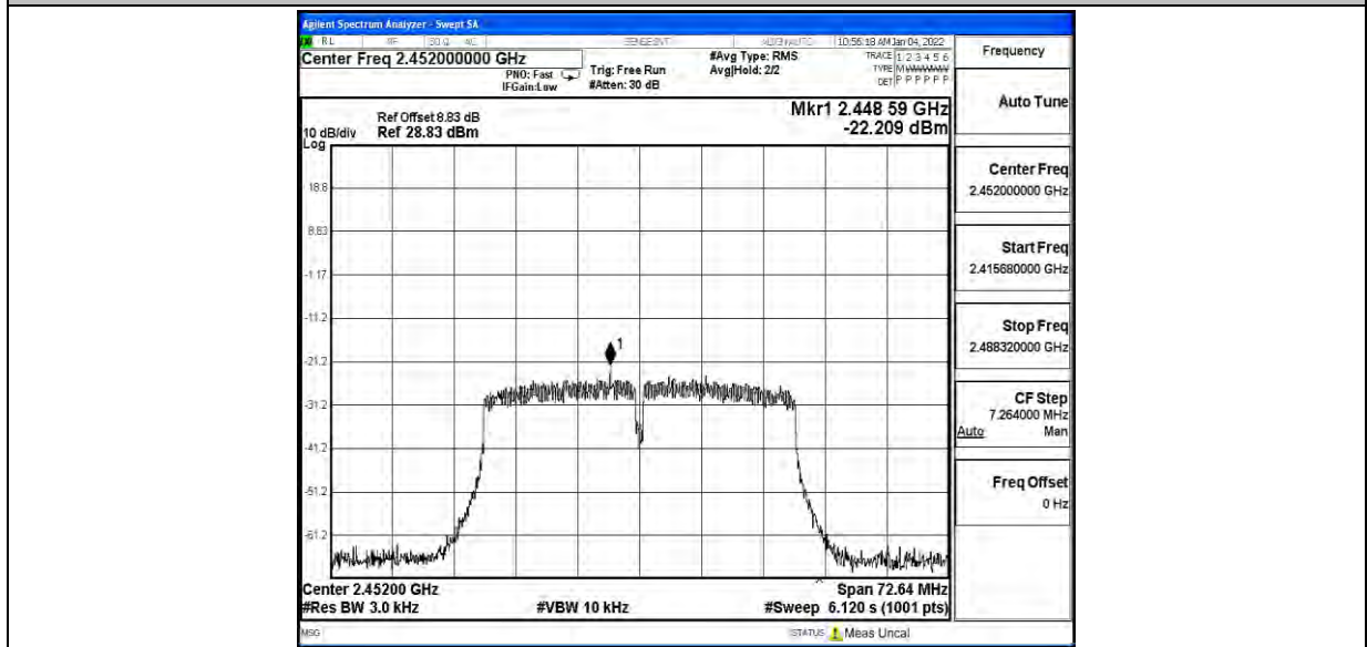
11N40SISO_Ant0_2452
