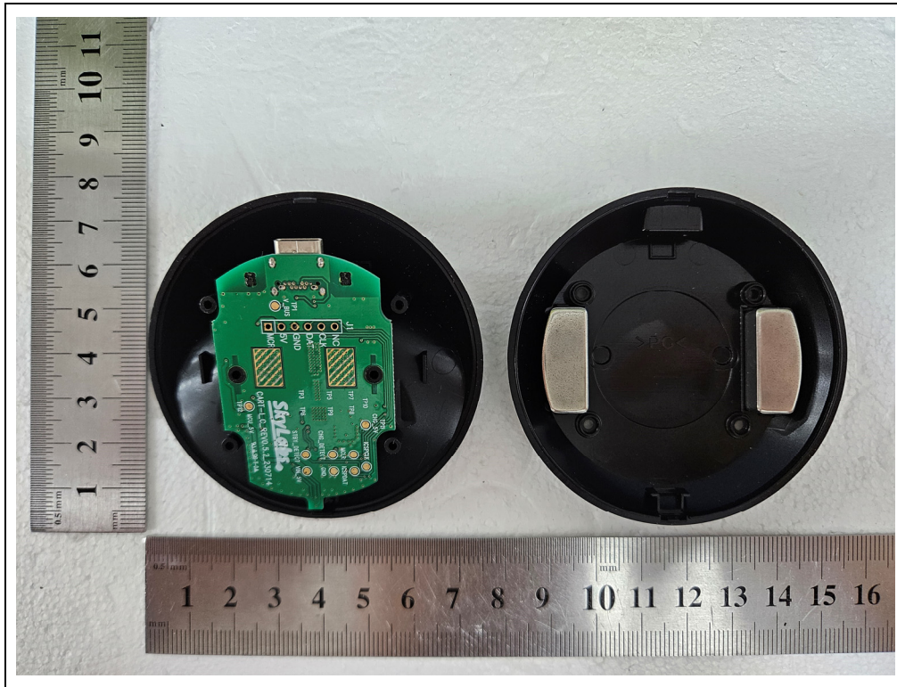
<PCB>
