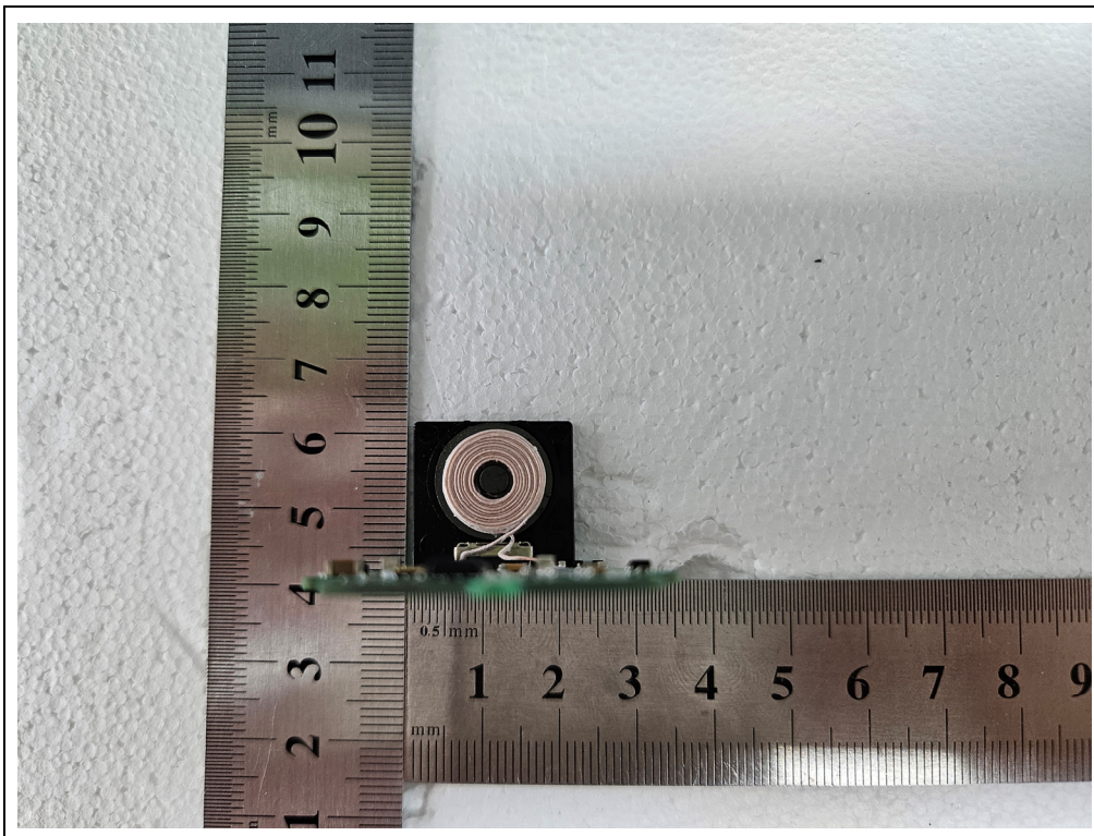
<ANT>
