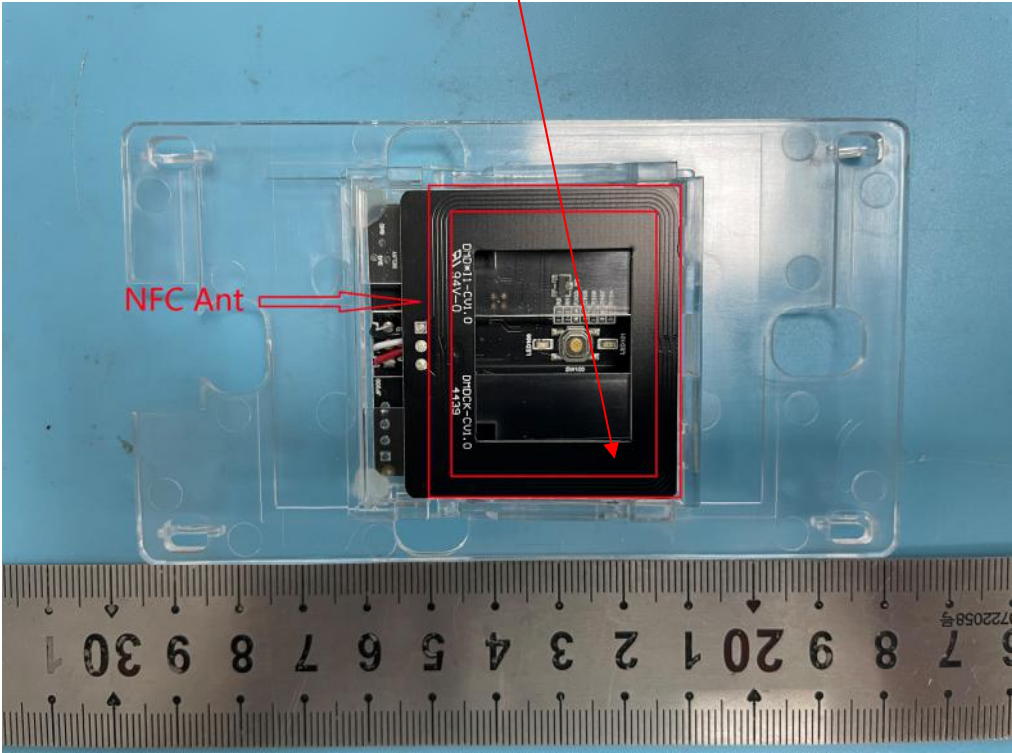
NFC Antenna
