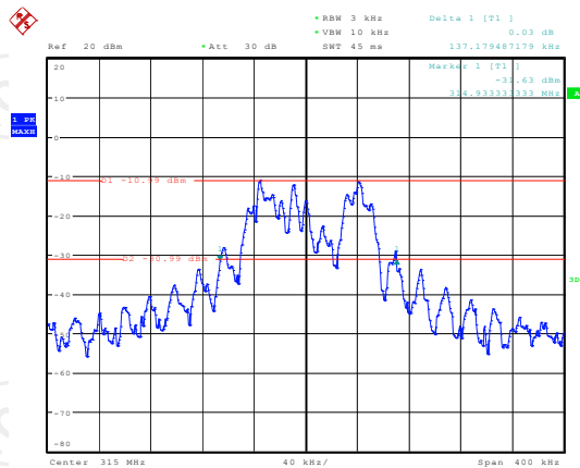
315MHz
