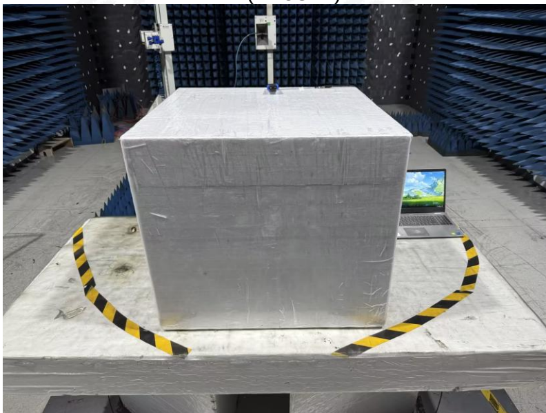
RE (1-18GHz)
