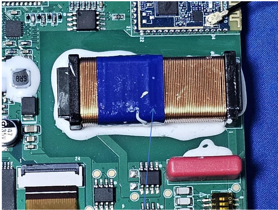
125K ANT
