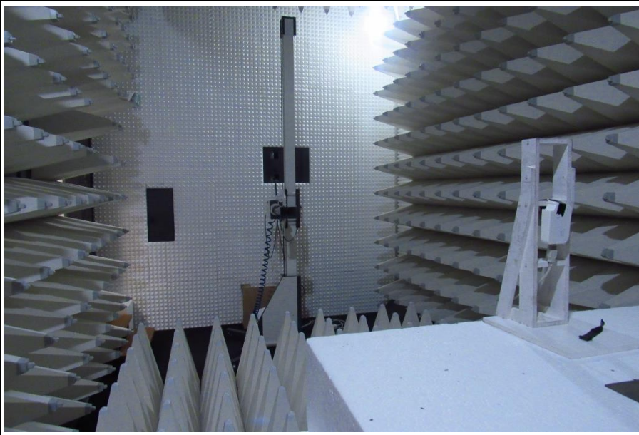
6G5-18G_2
