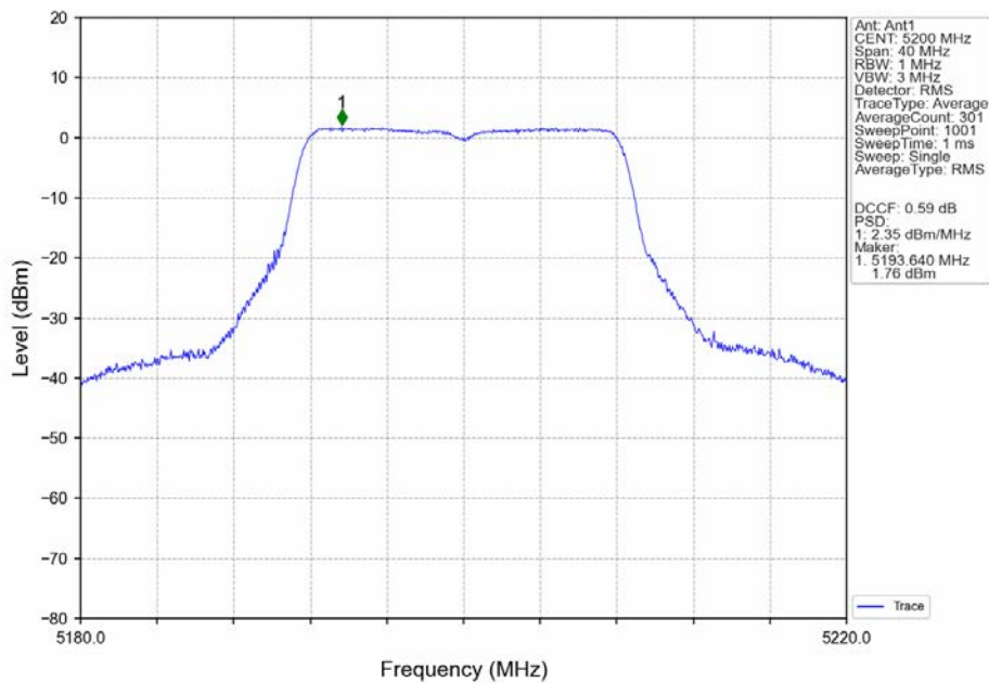
802.11a_MCH_5200MHz_Ant1_NTNV
