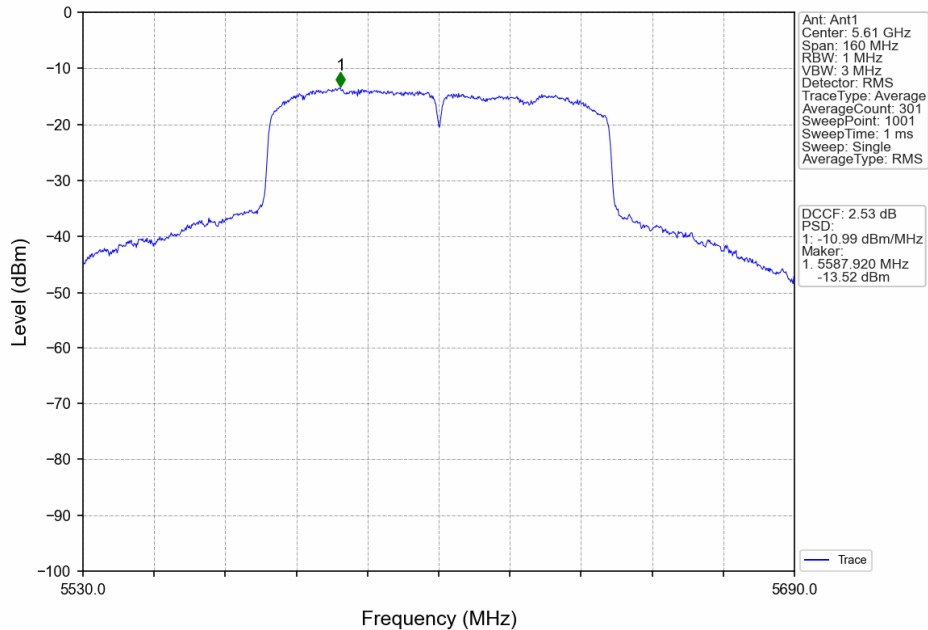
802.11ac(VHT80)_HCH_5610MHz_Ant1_NTNV
