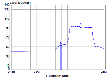
11n_HT(40M)_TX_CH_03_Horizontal-Avg
