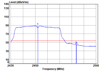
11n_HT(40M)_TX_CH_09_Vertical-Avg
