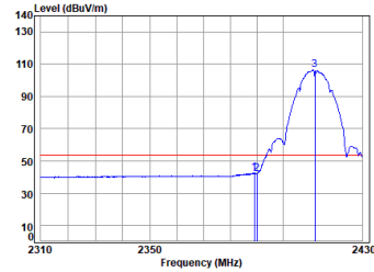
11b_TX_CH_01_Horizontal-Avg
