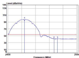
11b_TX_CH_11_Vertical-Avg
