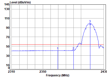
11b_TX_CH_01_Vertical-Avg
