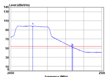
11n_HT(20M)_TX_CH_11_Horizontal-Avg
