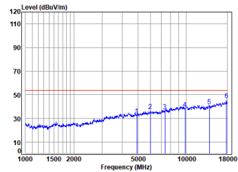
11n_HT(20M)_TX_CH_11_Horizontal-Avg
