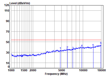
11n_HT(20M)_TX_CH_01_Horizontal-Avg
