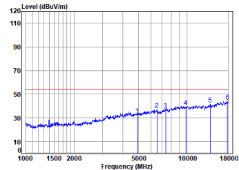
11n_HT(20M)_TX_CH_11_Vertical-Avg
