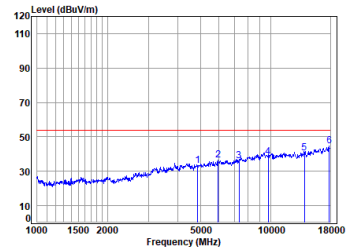
11n_HT(20M)_TX_CH_06_Vertical-Avg
