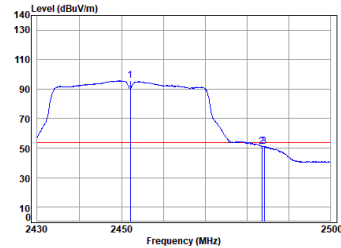
11n_HT(40M)_TX_CH_09_Horizontal-Avg
