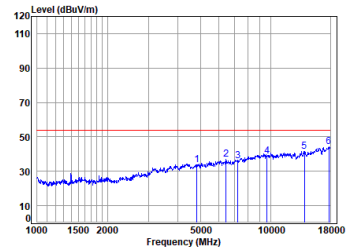
11n_HT(20M)_TX_CH_01_Vertical-Avg
