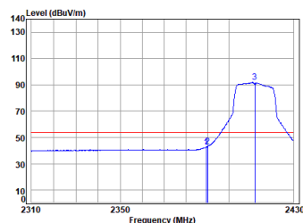
11n_HT(20M)_TX_CH_01_Vertical-Avg
