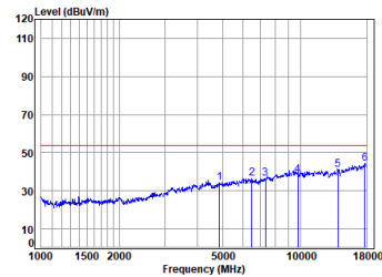
11b_TX_CH_06_Horizontal-Avg
