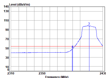
11n_HT(20M)_TX_CH_01_Horizontal-Avg
