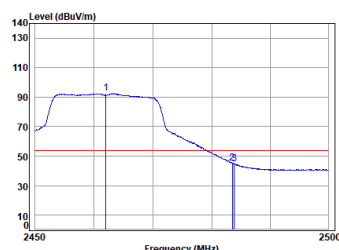
11n_HT(20M)_TX_CH_11_Vertical-Avg
