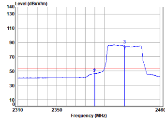
11n_HT(40M)_TX_CH_03_Vertical-Avg
