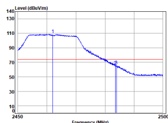
11n_HT(20M)_TX_CH_11_Horizontal-Peak
