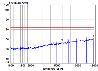
11n_HT(20M)_TX_CH_11_Horizontal-Peak
