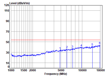
11n_HT(20M)_TX_CH_06_Horizontal-Avg
