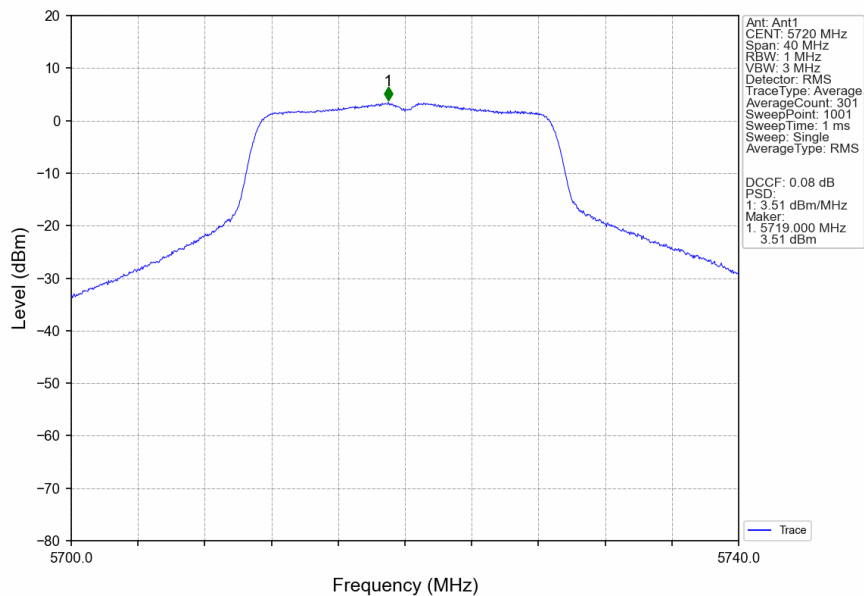
802.11ac(VHT20)_HCH_5720MHz_Ant1_NTNV
