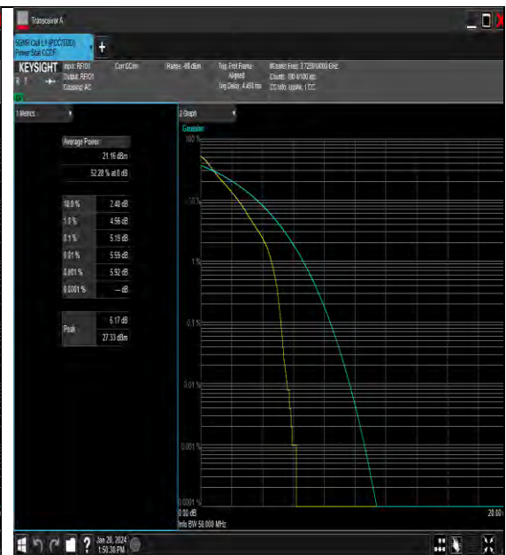
NTNV_N77-3700-3980_PC3_30_50_L_TID1_#1
