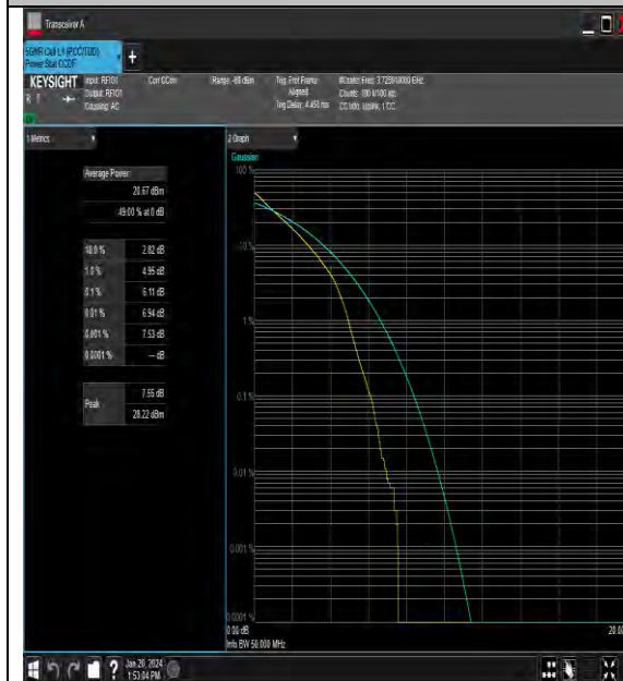
NTNV_N77-3700-3980_PC3_30_50_L_TID2_#1
