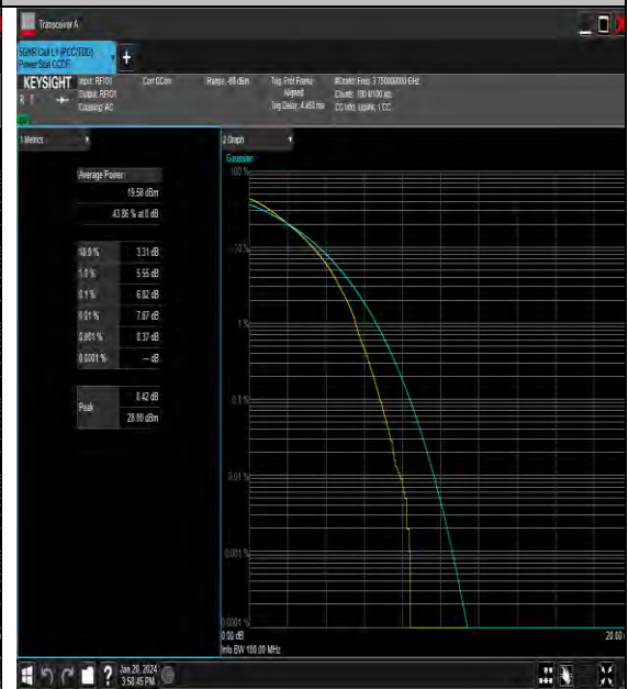
NTNV_N77-3700-3980_PC3_30_100_L_TID4_#1
