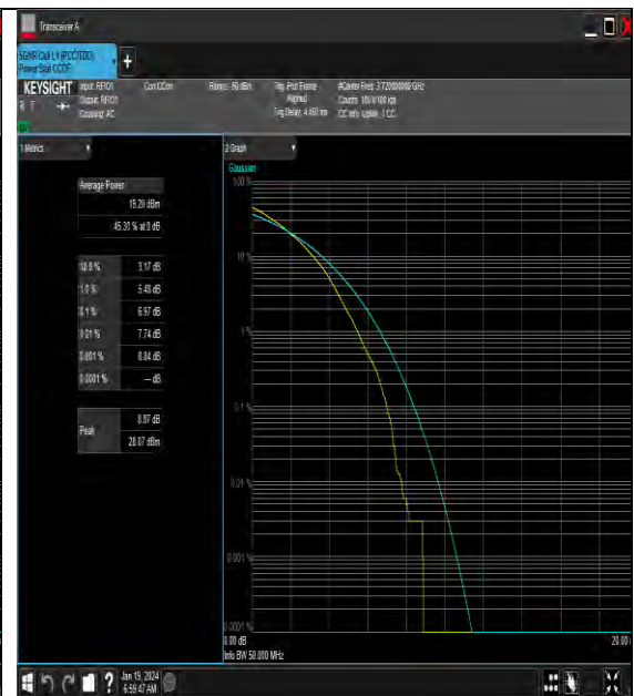
NTNV_N77-3700-3980_PC3_30_40_L_TID4_#1
