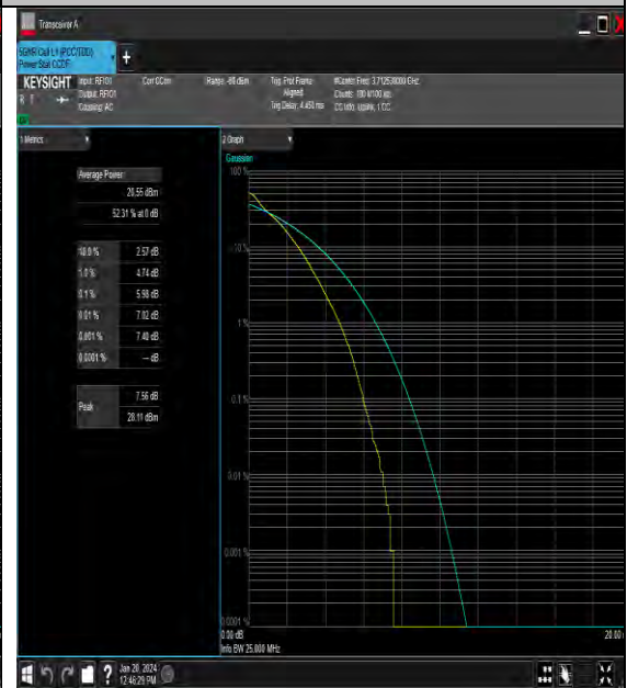
NTNV_N77-3700-3980_PC3_30_25_L_TID2_#1
