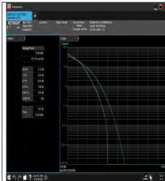
NTNV_N77-3700-3980_PC3_30_40_L_TID3_#1
