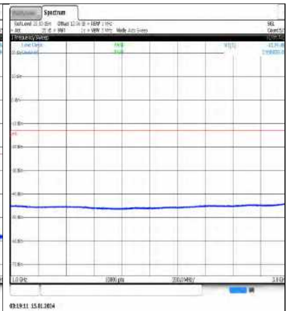
NTNV_N77-3450- 3550_PC3_30_20_L_TID5_NS_01_1000_3000_# 1
