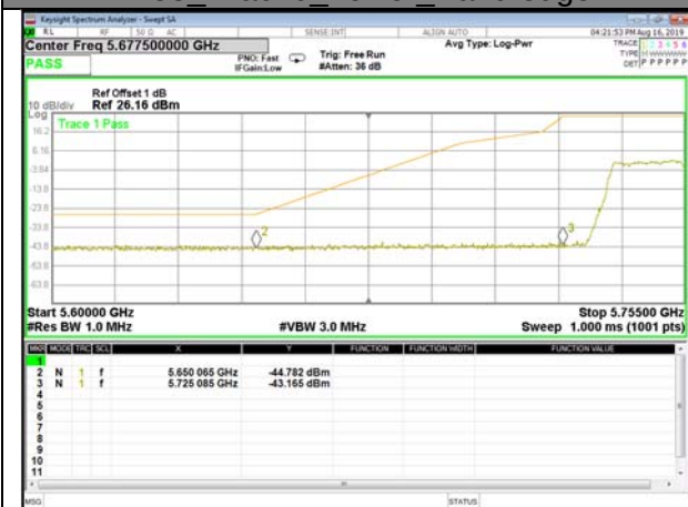
W58_11ac40_Lower_Band edge
