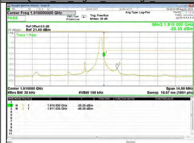
QPSK_3M_Higher_Band edge_1-RB
