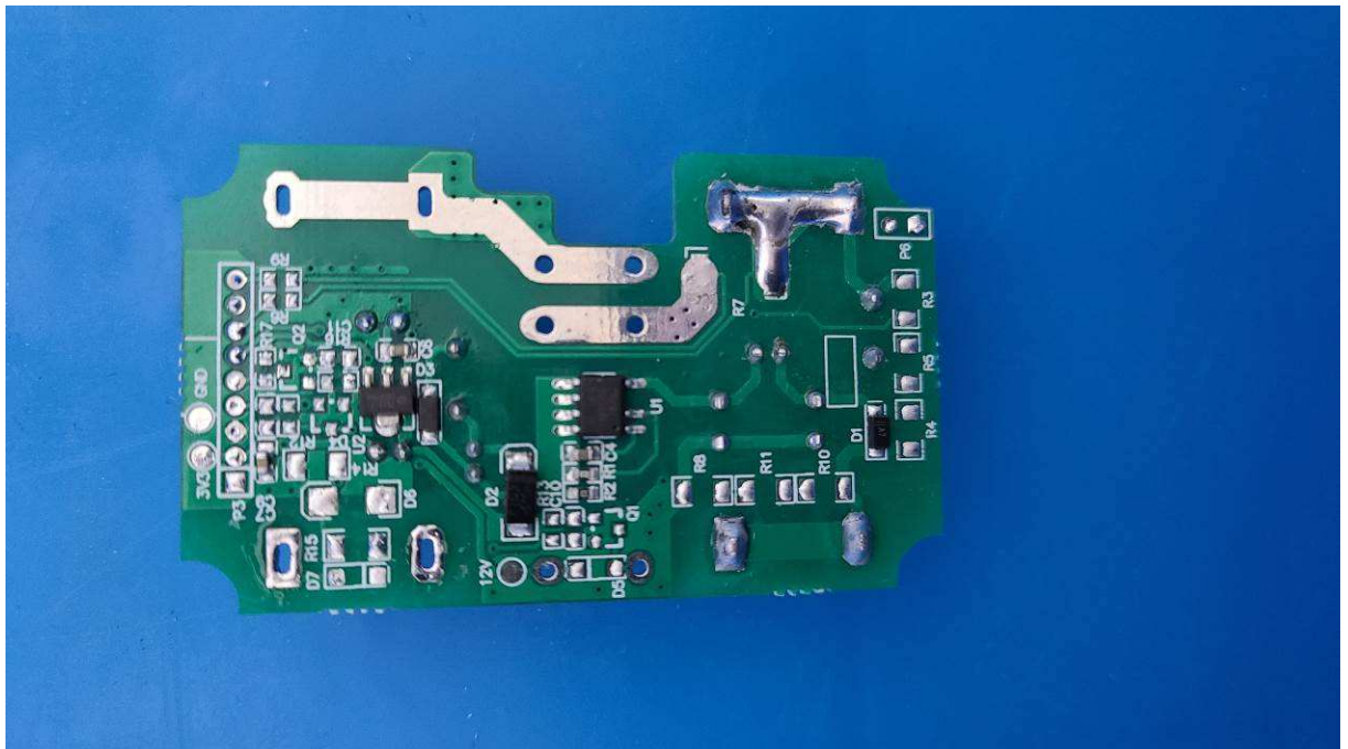
(10) EUT Photo
