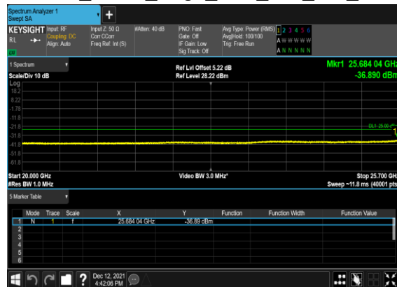
OFDM BPSK Edge 1RB Left Mid CH
