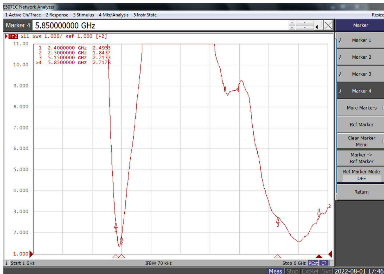
ANT24# VSWR
