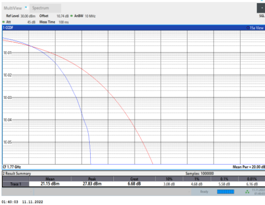
Band66-20MHz-QPSK-132572-100RB#0
