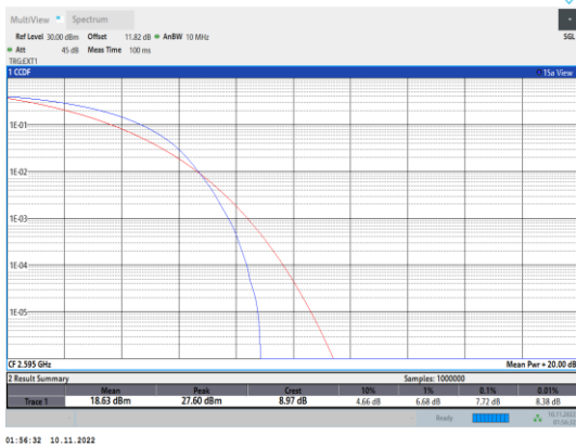
Band41-20MHz-QPSK-40640-100RB#0
