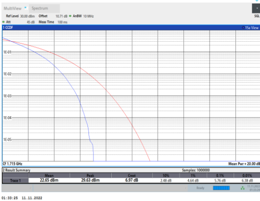
Band66-10MHz-QPSK-132022-50RB#0
