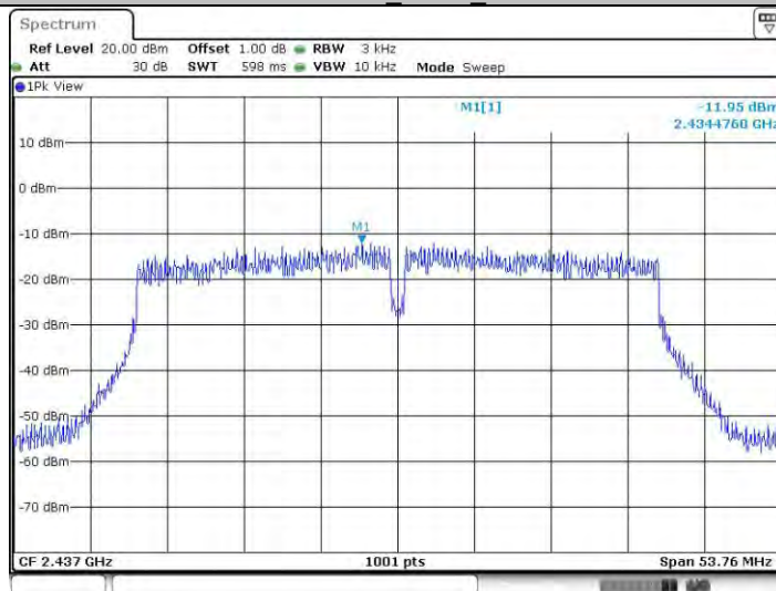
11n40SISO_Ant22_2437
