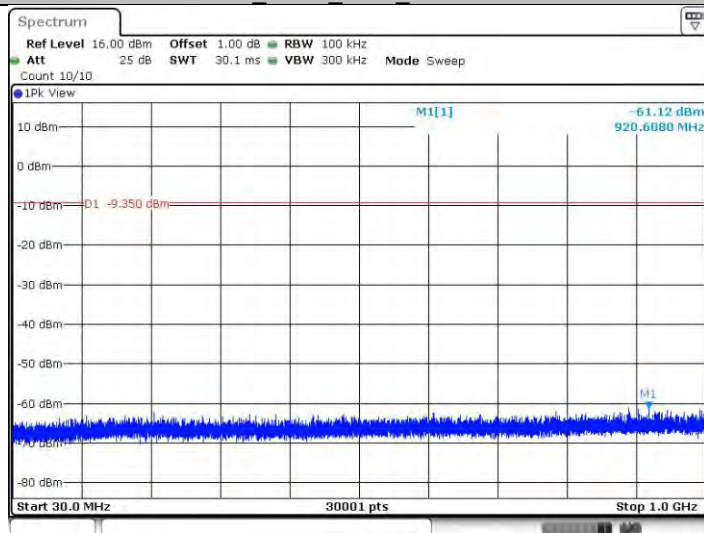
11b_Ant22_2462_30~1000
