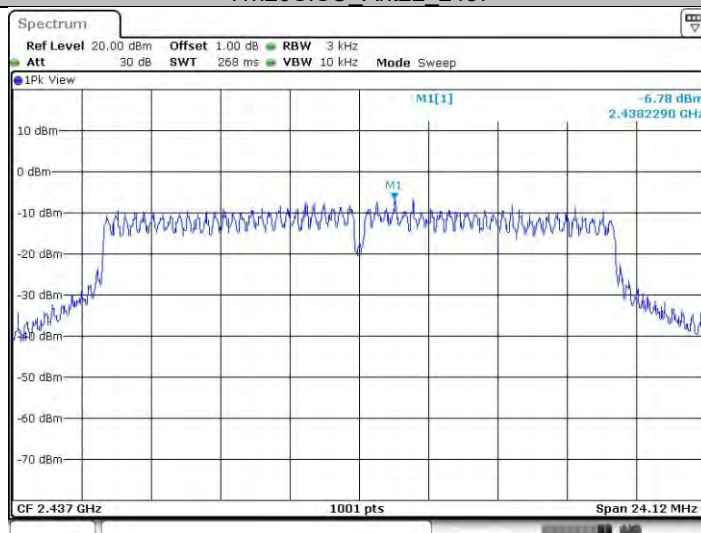
11n20SISO_Ant22_2437
