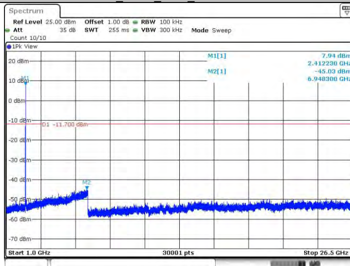
11b_Ant22_2412_1000~26500
