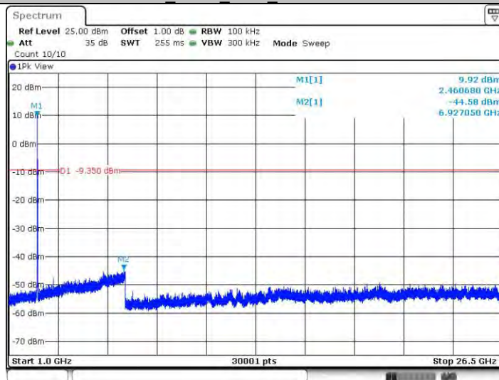
11b_Ant22_2462_1000~26500
