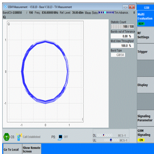
GSM850-190-5
