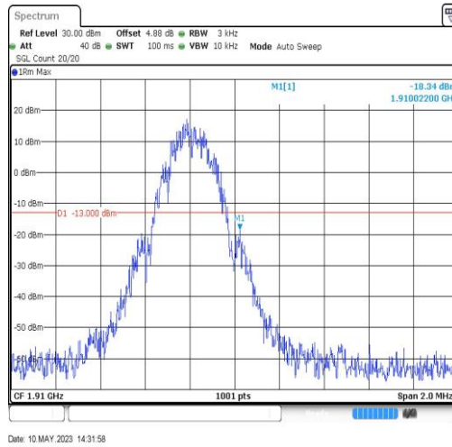
GSM1900-810-0-1910.02
