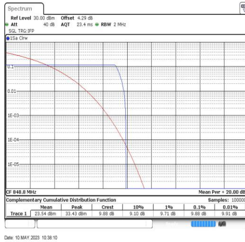
GSM850-251-5
