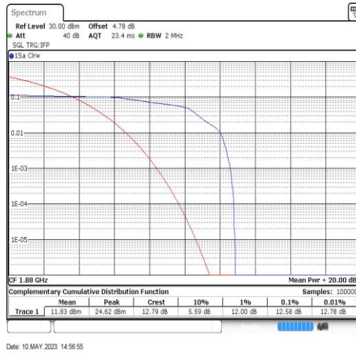
EGPRS1900-661-2
