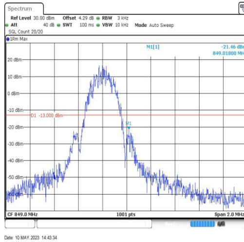
EGPRS850-251-8-849.02
