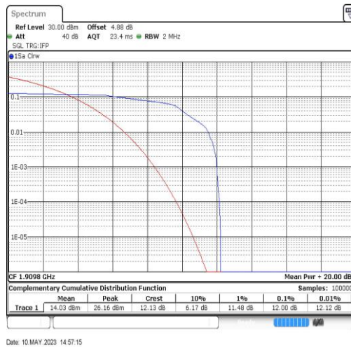
EGPRS1900-810-2
