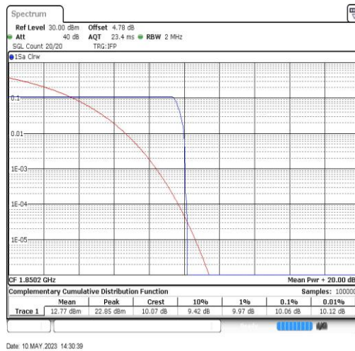
GSM1900-512-0
