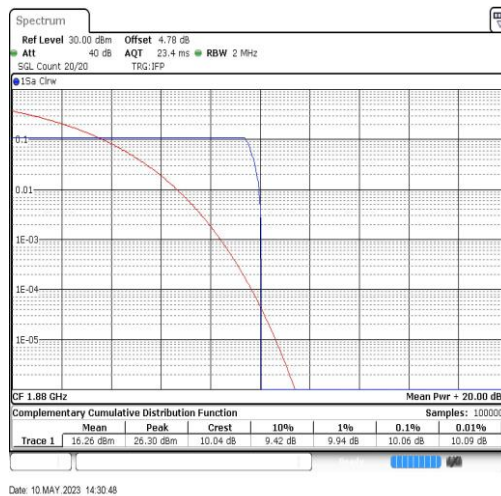
GSM1900-661-0
