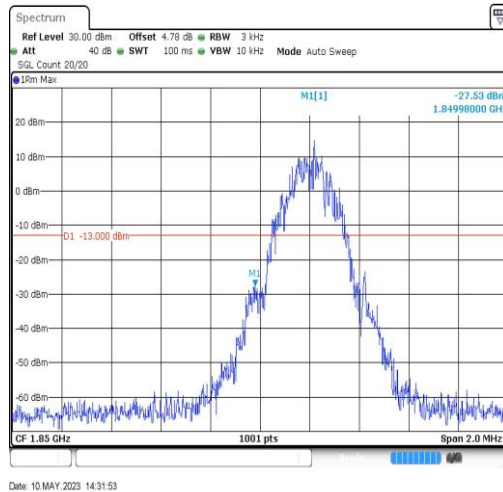
GSM1900-512-0-1849.98
