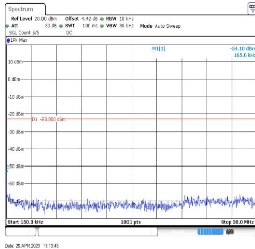
Band26-10MHz-QPSK-26740-1RB#0-Range2:0.15~30MHz
