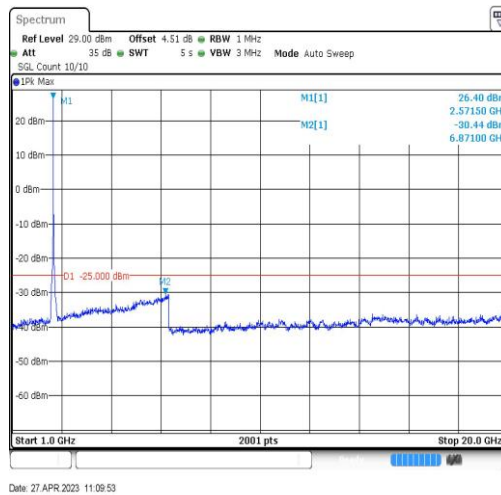
Band38-20MHz-QPSK-37850-1RB#0-Range4:1000~20000MHz
