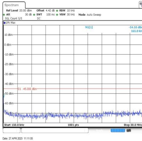
Band38-20MHz-QPSK-38000-1RB#0-Range2:0.15~30MHz
