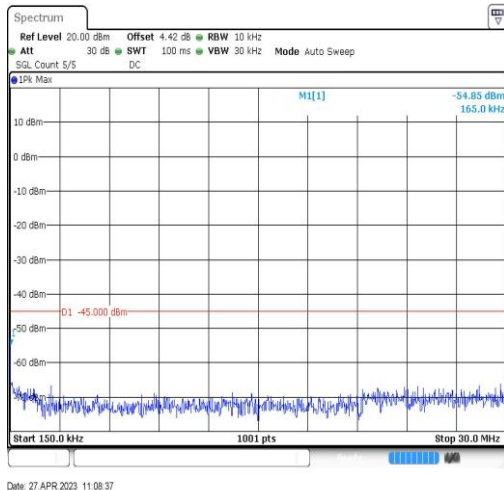
Band38-20MHz-QPSK-37850-1RB#0-Range2:0.15~30MHz
