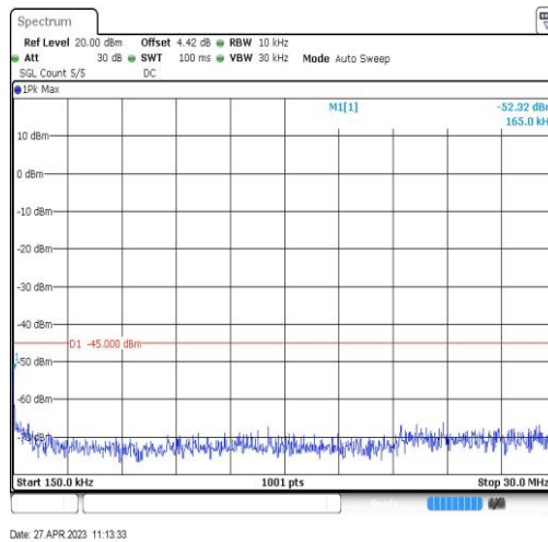
Band38-20MHz-QPSK-38150-1RB#0-Range2:0.15~30MHz
