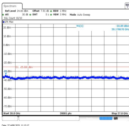
Band38-20MHz-QPSK-38000-1RB#0-Range5:20000~27000MHz
