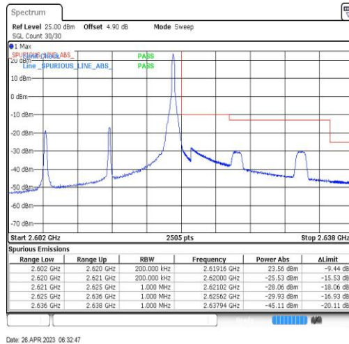
Band38-15MHz-QPSK-38175-1RB#74
