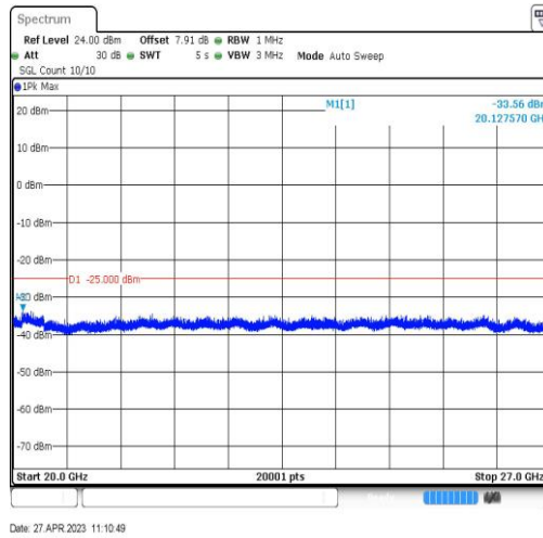
Band38-20MHz-QPSK-37850-1RB#0-Range5:20000~27000MHz
