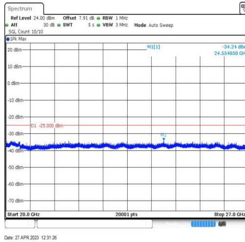
Band41-20MHz-QPSK-39750-1RB#0-Range5:20000~27000MHz
