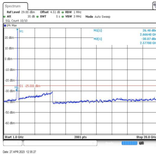
Band41-20MHz-QPSK-41490-1RB#0-Range4:1000~20000MHz
