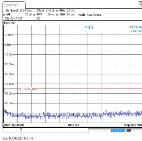
Band41-20MHz-QPSK-40620-1RB#0-Range2:0.15~30MHz
