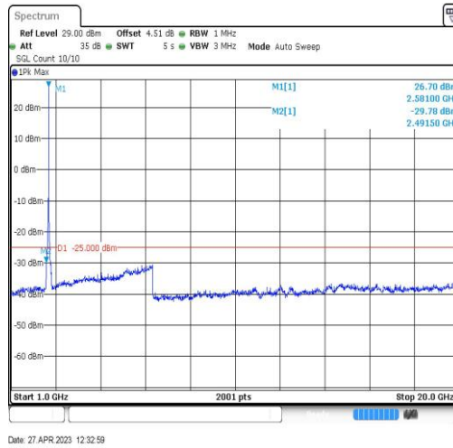
Band41-20MHz-QPSK-40620-1RB#0-Range4:1000~20000MHz
