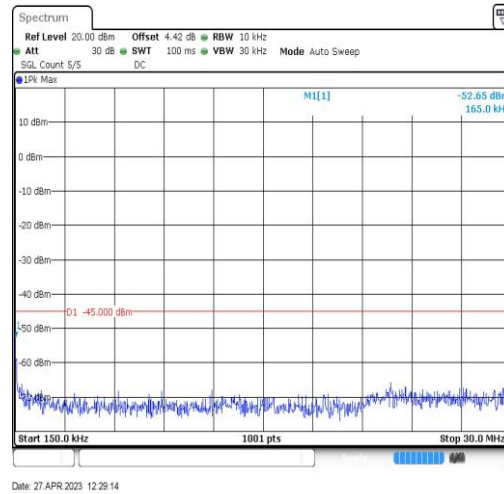
Band41-20MHz-QPSK-39750-1RB#0-Range2:0.15~30MHz
