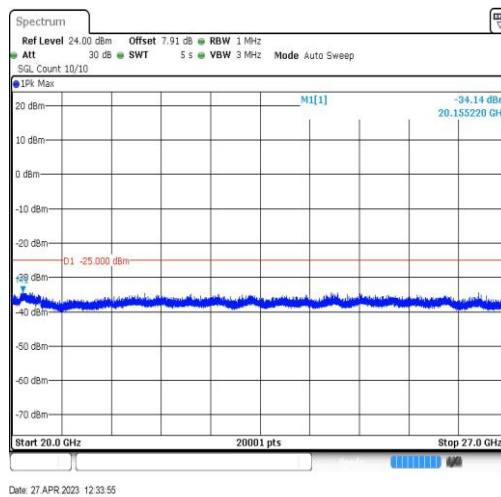
Band41-20MHz-QPSK-40620-1RB#0-Range5:20000~27000MHz
