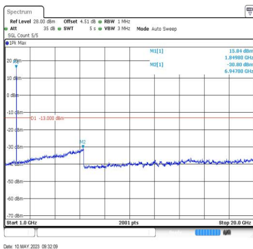
BandII-9262-1000~20000MHz-6947
