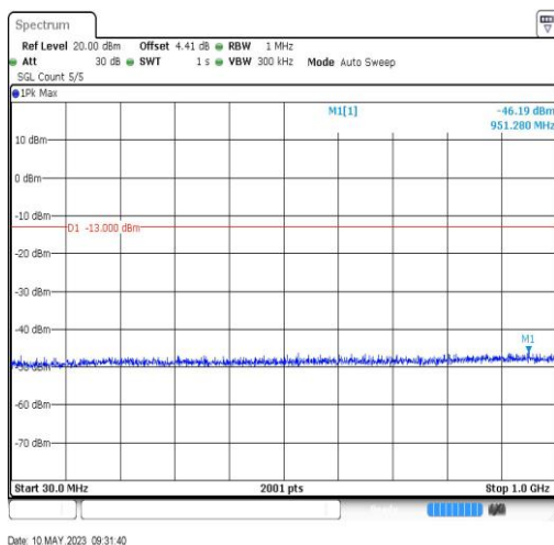
BandII-9262-30~1000MHz-951.28
