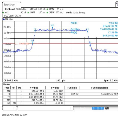
Band5-3MHz-QPSK-20635-15RB#0-2.697
