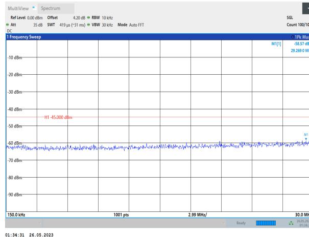
Band38-20MHz-QPSK-37850-1RB#0-Range2:0.15~30MHz
