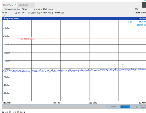
Band66-20MHz-QPSK-132072-1RB#0-Range2:0.15~30MHz
