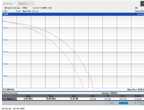
38-38-20MHz-20MHz-QPSK-QPSK-37901-38099-100RB#0-100RB#0
