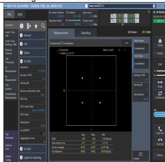
NTNV,N66,_PC3,_15,40,M,TID6,#1
