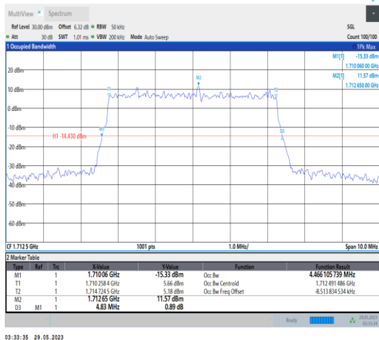
NTVN_N66_PC3_15_5_L_TID5_Ant1#1
