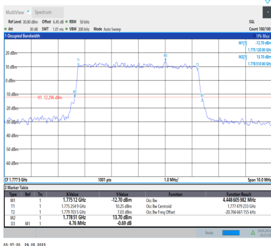
NTNV_N66_PC3_15_5_H_TID1_Ant1#1
