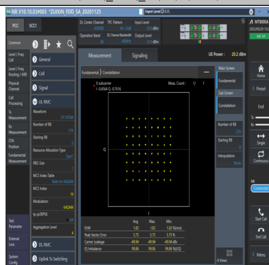
NTNV,N66,_PC3,_15,40,M,TID8,#1
