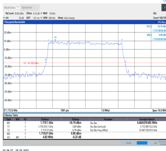
NTVN_N66_PC3_15_5_L_TID8_Ant1#1
