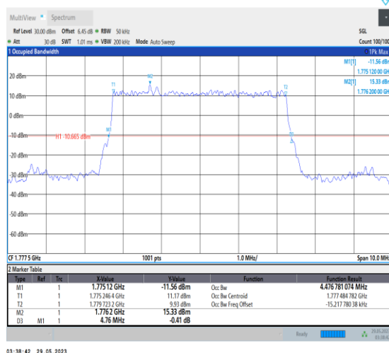
NTNV_N66_PC3_15_5_H_TID2_Ant1#1
