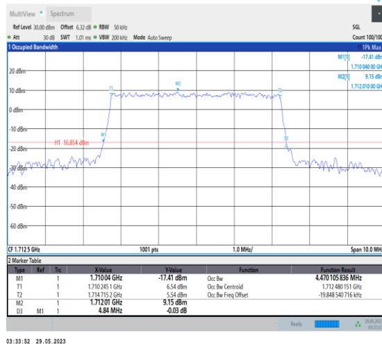
NTVN_N66_PC3_15_5_L_TID6_Ant1#1
