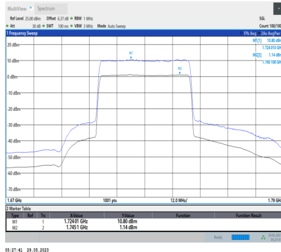
NTNV_N66_PC3_15_40_L_TID2_#1
