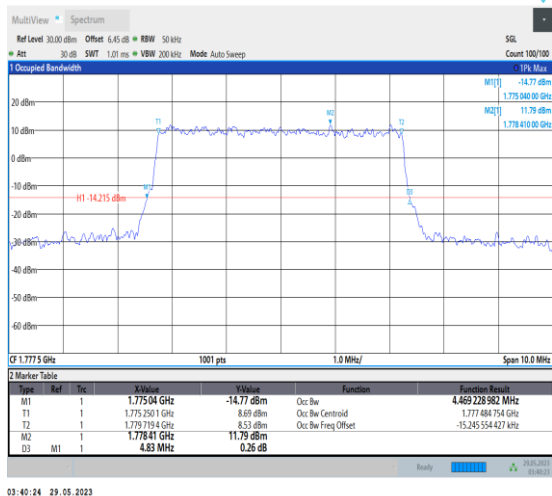
NTNV_N66_PC3_15_5_H_TID3_Ant1#1
