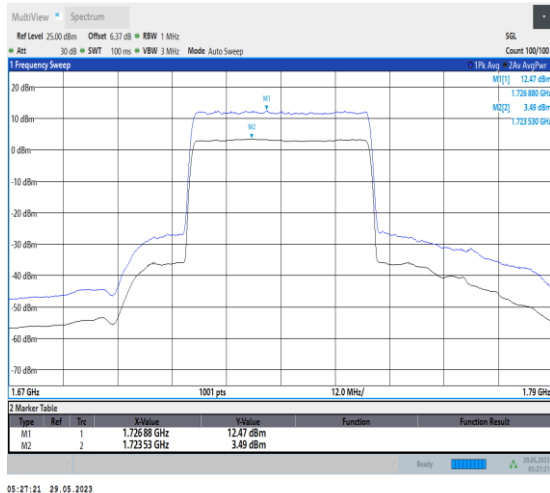
NTNV_N66_PC3_15_40_L_TID1_#1
