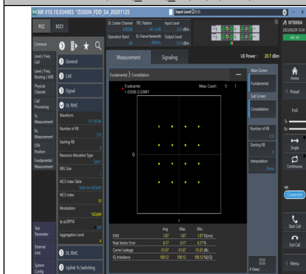
NTNV,N66,_PC3,_15,40,M,TID7,#1
