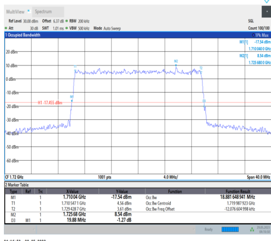
NTNV_N66_PC3_15_20_L_TID9_Ant1#1
