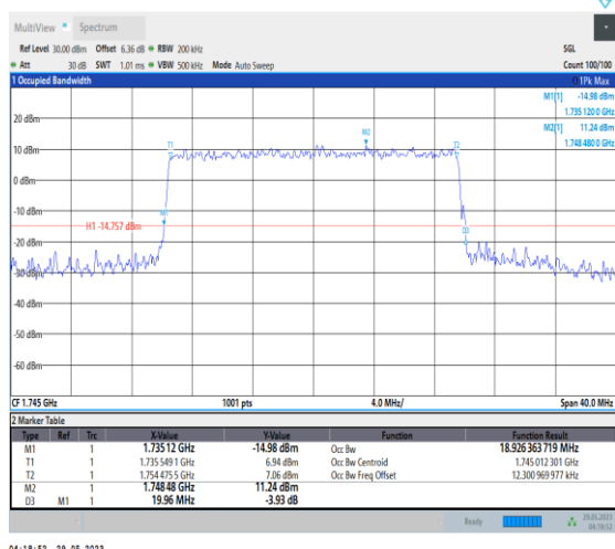
NTNV_N66_PC3_15_20_M_TID6_Ant1#1
