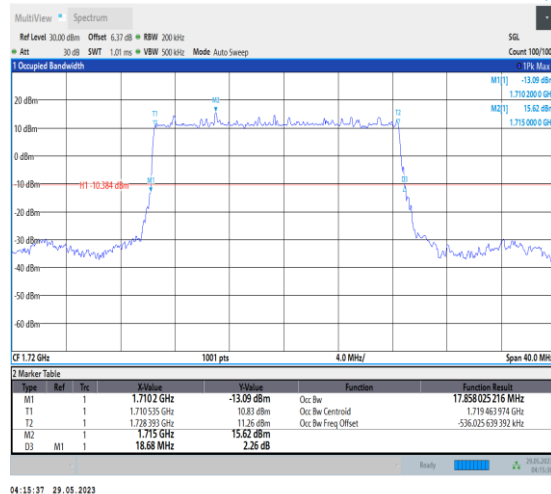
NTNV_N66_PC3_15_20_L_TID2_Ant1#1
