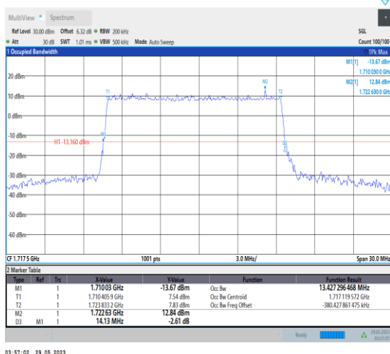
NTNV_N66_PC3_15_15_L_TID5_Ant1#1
