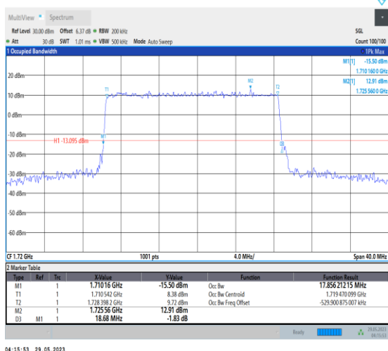
NTNV_N66_PC3_15_20_L_TID3_Ant1#1
