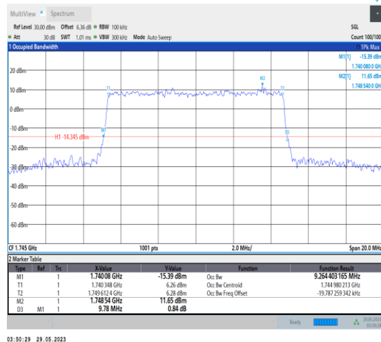
NTNV_N66_PC3_15_10_M_TID6_Ant1#1
