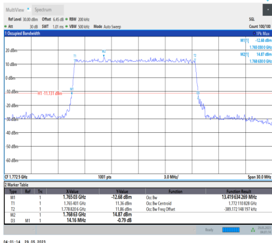
NTNV_N66_PC3_15_15_H_TID1_Ant1#1
