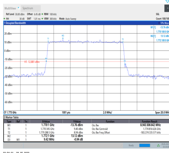
NTNV_N66_PC3_15_10_H_TID3_Ant1#1
