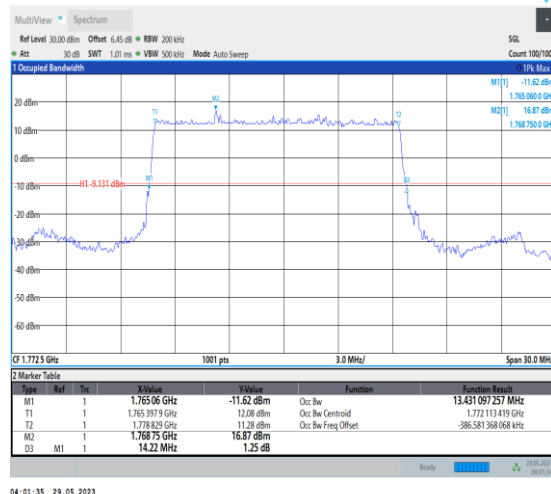
NTNV_N66_PC3_15_15_H_TID2_Ant1#1
