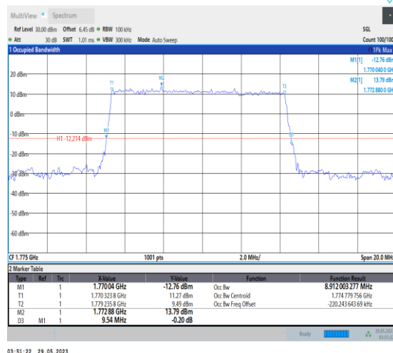
NTNV_N66_PC3_15_10_H_TID1_Ant1#1
