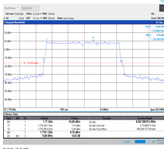
NTNV_N66_PC3_15_10_L_TID5_Ant1#1
