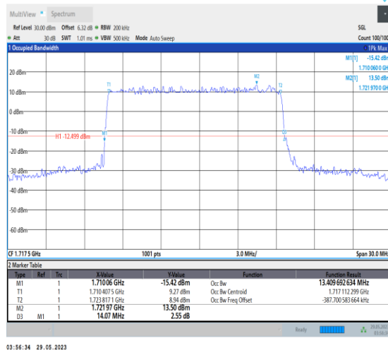
NTNV_N66_PC3_15_15_L_TID4_Ant1#1
