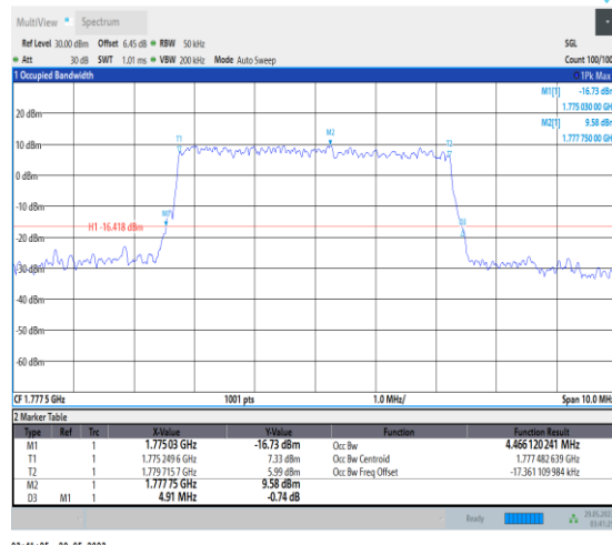
NTVN_N66_PC3_15_5_H_TID8_Ant1#1
