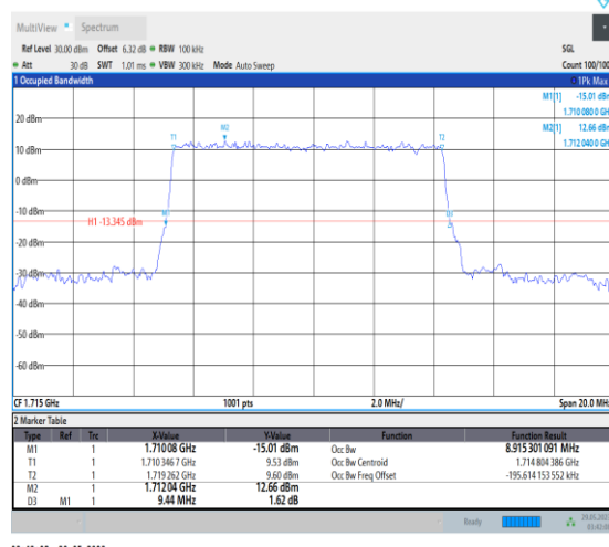
NTVN_N66_PC3_15_10_L_TID1_Ant1#1
