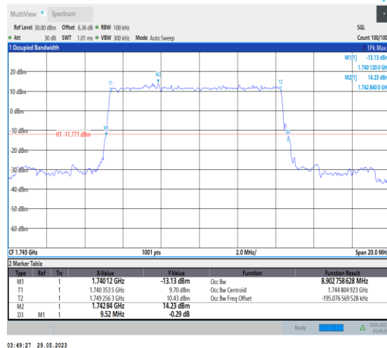
NTNV_N66_PC3_15_10_M_TID2_Ant1#1
