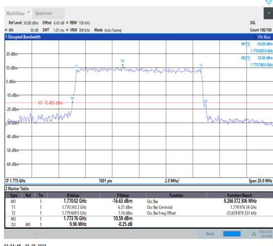
NTNV_N66_PC3_15_10_H_TID6_Ant1#1
