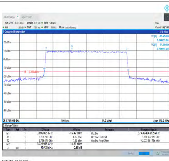
1-N78-3700-3800-PC3-30-70-L-7-CP-16QAM-Outer_Full-189@0-Ant1-67.435-70.420-≤70-PASS
