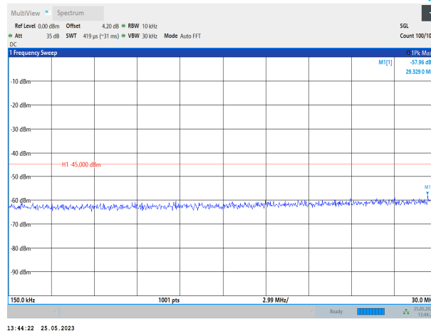
Band7-20MHz-QPSK-20850-1RB#0-Range2:0.15~30MHz
