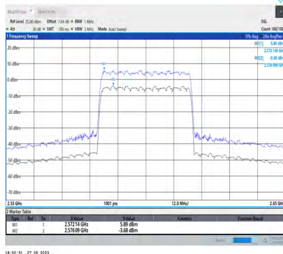
1-N38-PC3-30-40-L-2-CP-256QAM-Outer_Full-106@ 0-9.57-100%-0.00-9.57-PASS≤13
