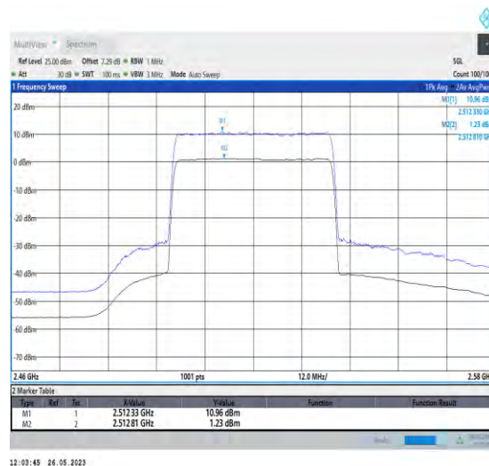
1-N7-PC3-15-40-L-2-CP-256QAM-Outer_Full-216@ 0-9.73-100%-0.00-9.73-PASS-≤13
