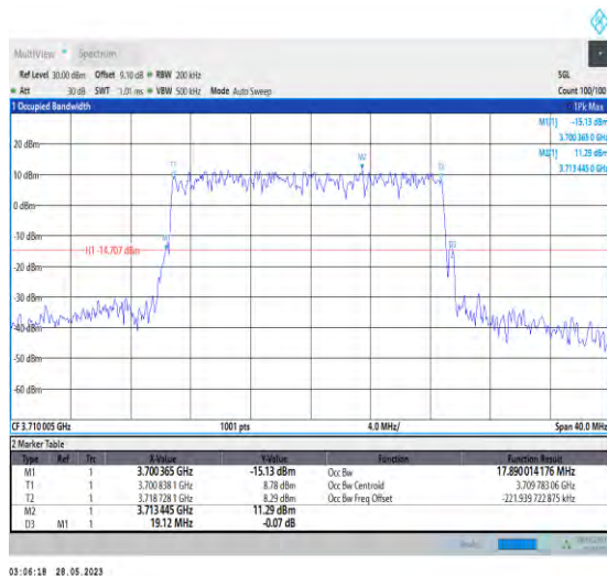
1-N77-3700-3980-PC3-30-20-L-3-DFT-16QAM-Out_ Full-50@0-17.89-19.120-≤20-PASS
