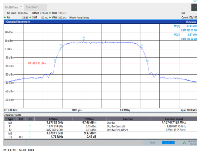
Band II-9400-4.76
