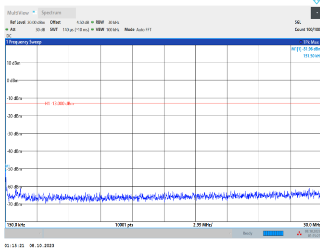
GSM850-128-0.15~30MHz
