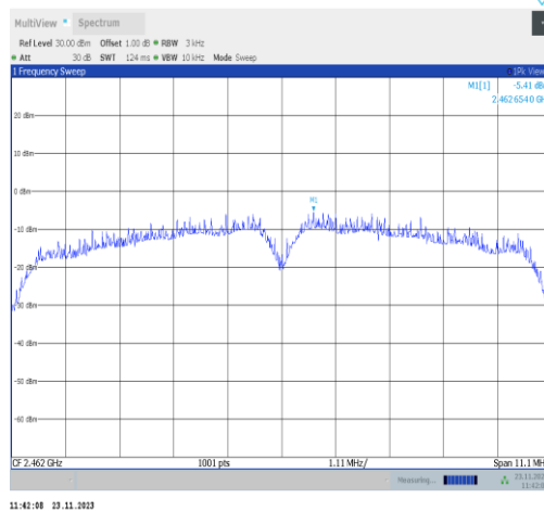
11b-CDD-Ant25-2462-PASS
