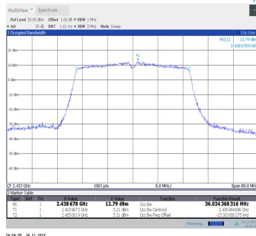
11VHT40MIMO-Ant25-2437
