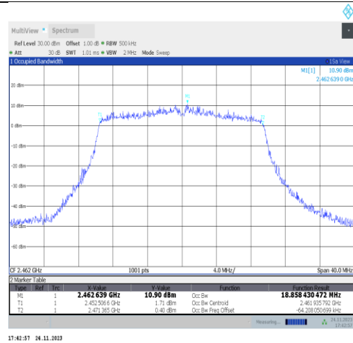
11ax20MIMO-Ant25-2462
