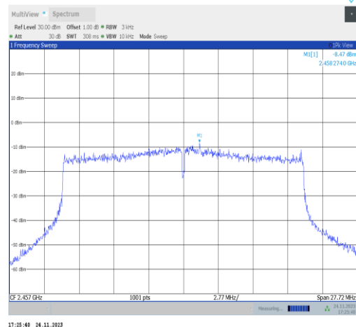
11ax20MIMO-Ant25-2457-PASS
