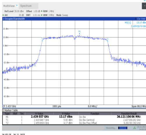
11VHT40MIMO-Ant22-2437
