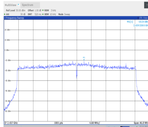
11ax40MIMO-Ant25-2437-PASS
