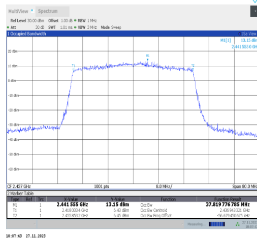
11ax40MIMO-Ant25-2437
