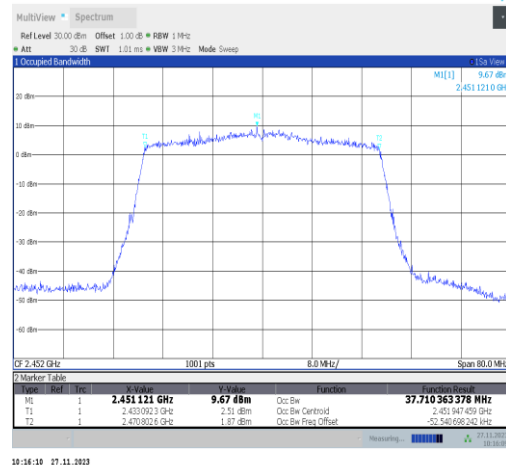
11ax40MIMO-Ant25-2452
