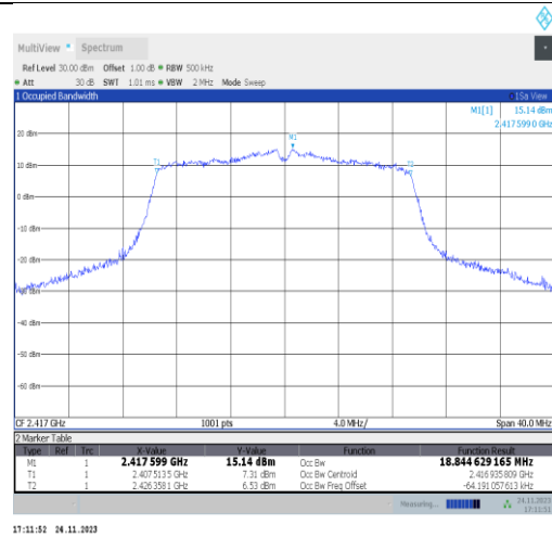
11ax20MIMO-Ant25-2417
