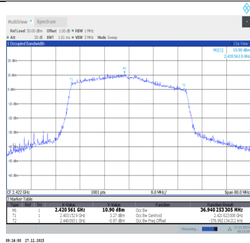
11ax40MIMO-Ant25-2422
