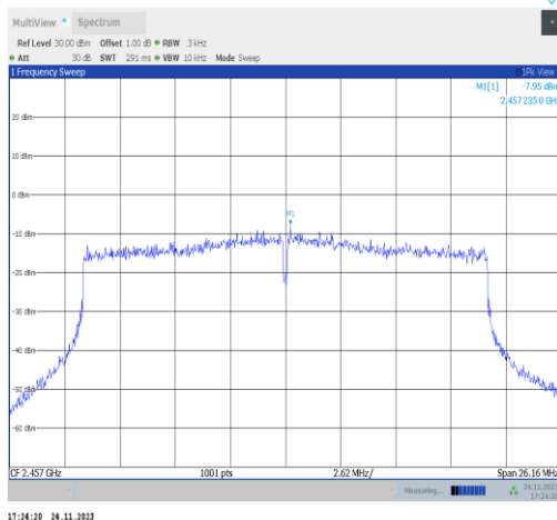
11ax20MIMO-Ant22-2457-PASS
