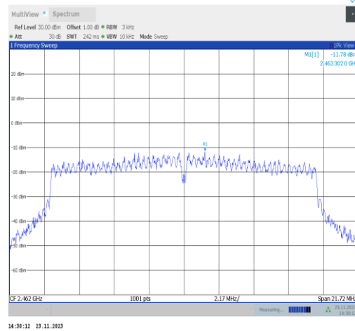
11g-CDD-Ant25-2462-PASS
