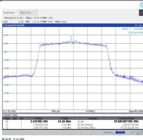
11ax40MIMO-Ant22-2427
