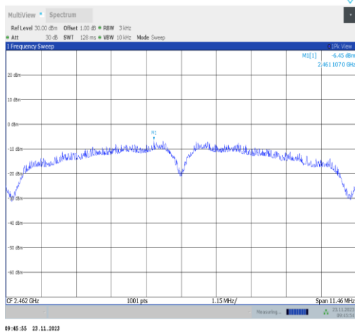
11b-CDD-Ant22-2462-PASS
