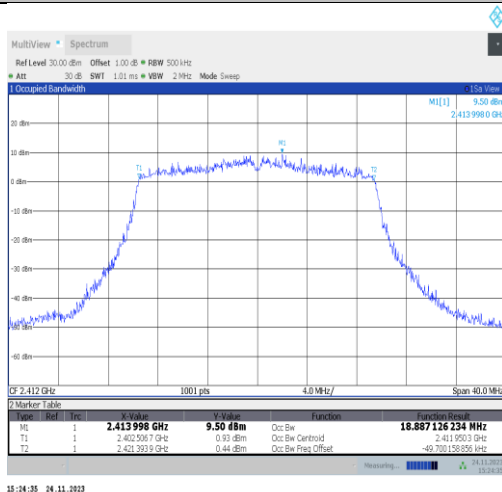
11ax20MIMO-Ant22-2412
