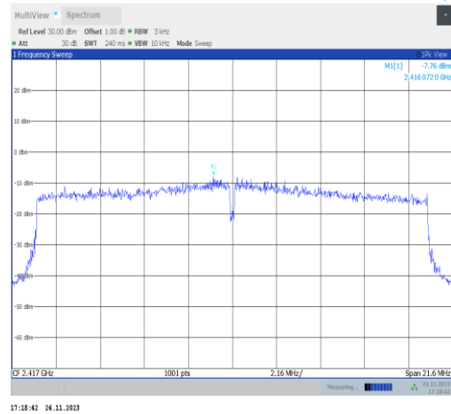
11ax20MIMO-Ant25-2417-PASS
