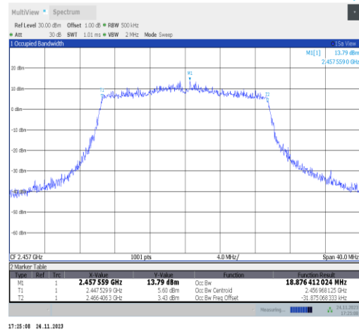
11ax20MIMO-Ant25-2457
