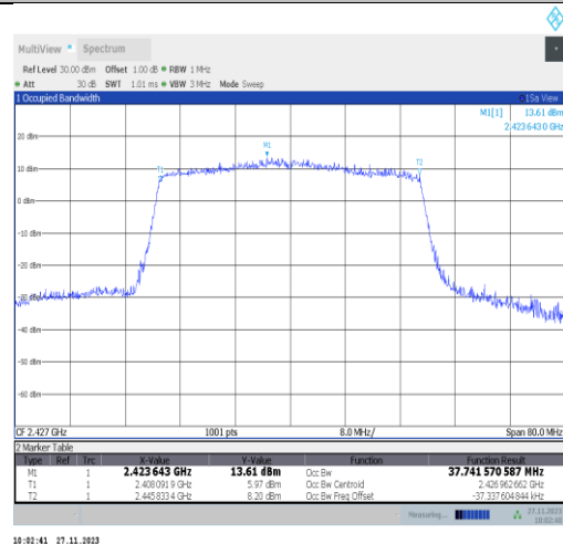
11ax40MIMO-Ant25-2427
