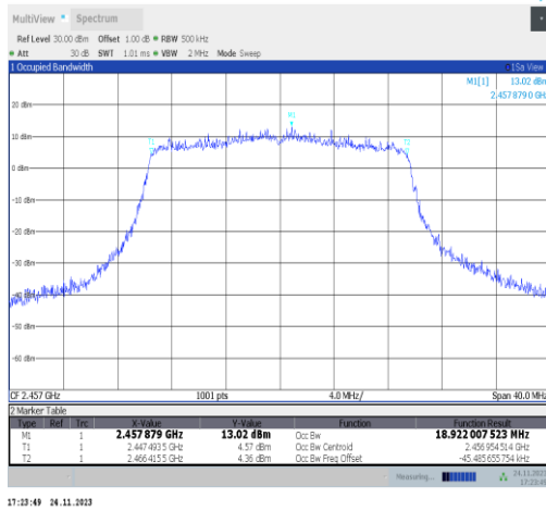
11ax20MIMO-Ant22-2457
