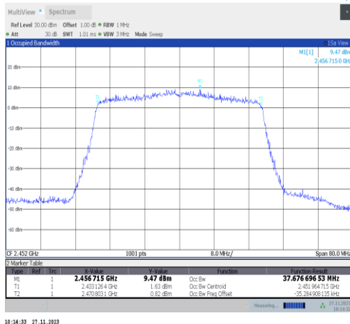
11ax40MIMO-Ant22-2452
