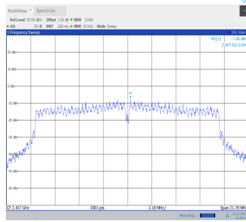
11g-CDD-Ant25-2457-PASS
