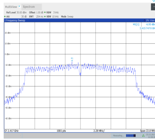
11g-CDD-Ant25-2417-PASS
