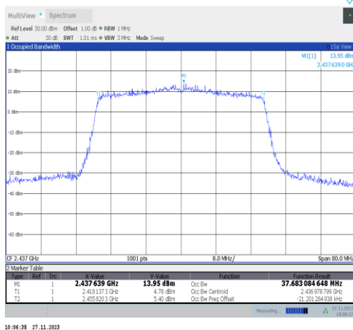
11ax40MIMO-Ant22-2437
