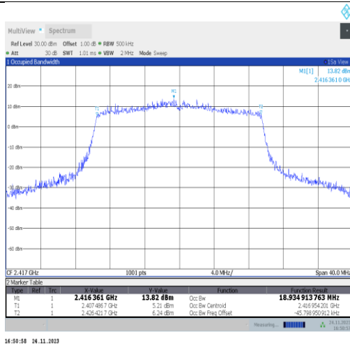
11ax20MIMO-Ant22-2417
