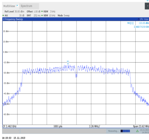
11g-CDD-Ant22-2462-PASS
