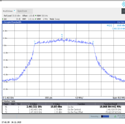
11ax20MIMO-Ant22-2462
