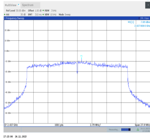
11ax20MIMO-Ant25-2437-PASS
