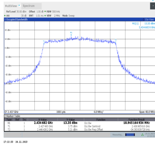
11ax20MIMO-Ant25-2437
