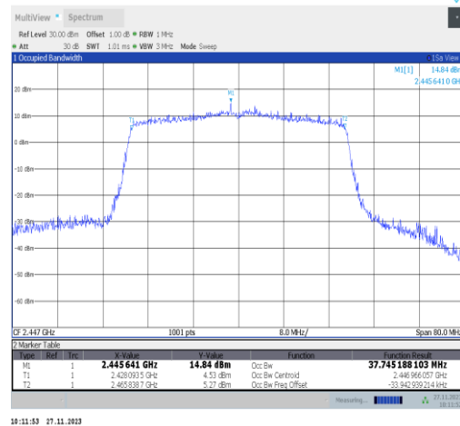
11ax40MIMO-Ant25-2447
