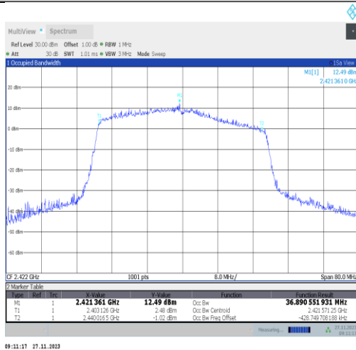
11ax40MIMO-Ant22-2422
