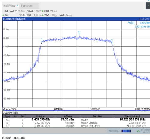
11ax20MIMO-Ant22-2437
