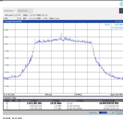
11ax20MIMO-Ant25-2412
