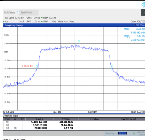
11ax20MIMO-Ant25-5500
