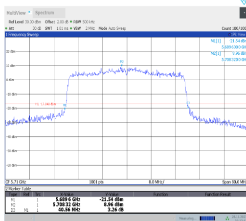
11ax40MIMO-Ant25-5710
