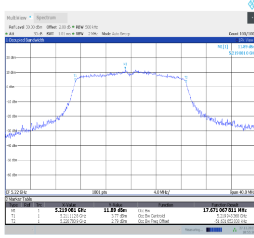
11n20MIMO-Ant25-5220
