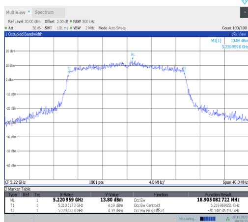
11ax20MIMO-Ant25-5220
