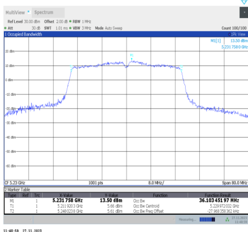
11n40MIMO-Ant22-5230
