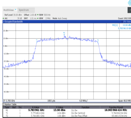
11ax20MIMO-Ant25-5785
