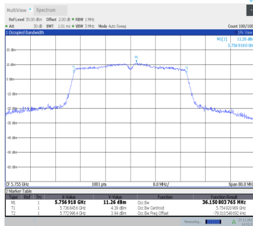
11n40MIMO-Ant25-5755
