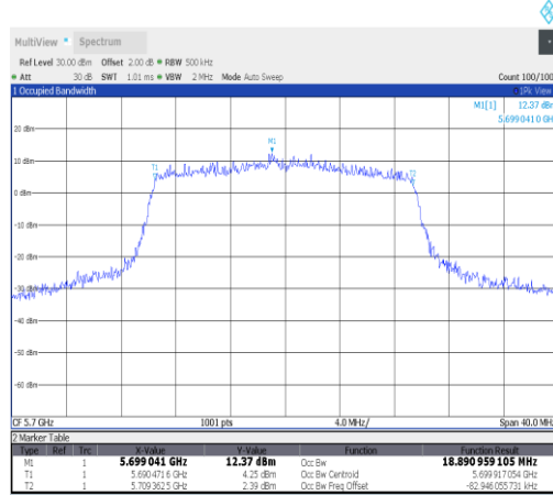
11ax20MIMO-Ant25-5700
