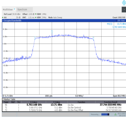
11ax40MIMO-Ant22-5710
