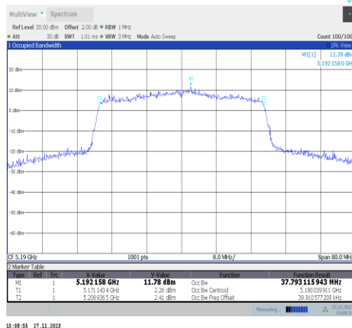
11ax40MIMO-Ant25-5190
