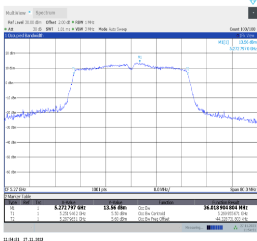
11n40MIMO-Ant22-5270
