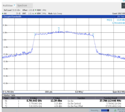
11ax40MIMO-Ant22-5795
