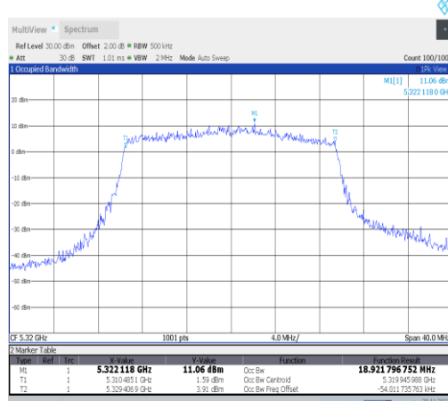
11ax20MIMO-Ant25-5320
