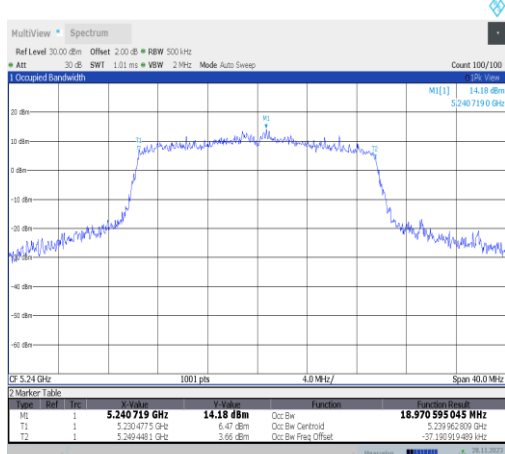
11ax20MIMO-Ant22-5240
