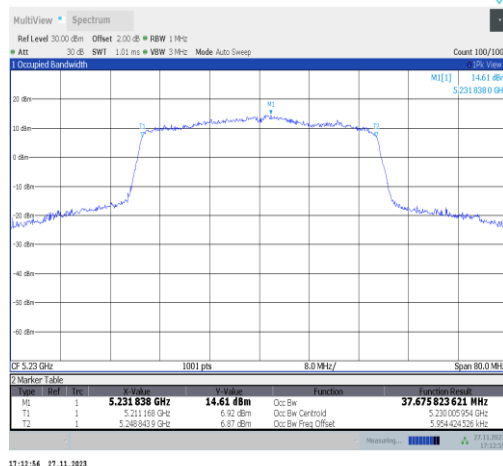
11ax40MIMO-Ant25-5230
