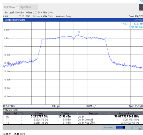
11n40MIMO-Ant25-5270
