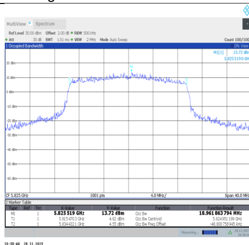
11ax20MIMO-Ant25-5825
