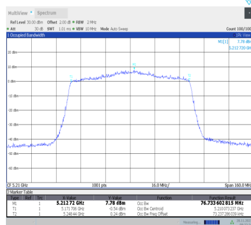
11ax80MIMO-Ant25-5210
