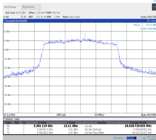
11ax20MIMO-Ant25-5300
