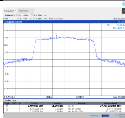
11ax40MIMO-Ant25-5755
