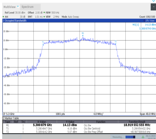
11ax20MIMO-Ant22-5300
