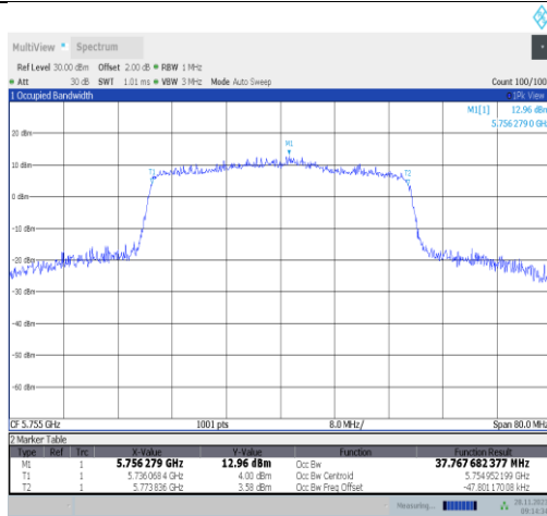
11ax40MIMO-Ant22-5755
