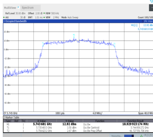
11ax20MIMO-Ant25-5745
