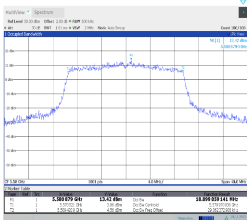
11ax20MIMO-Ant22-5580
