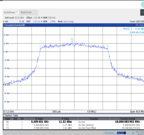
11ax20MIMO-Ant25-5500
