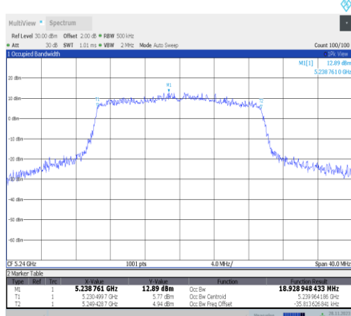
11ax20MIMO-Ant25-5240
