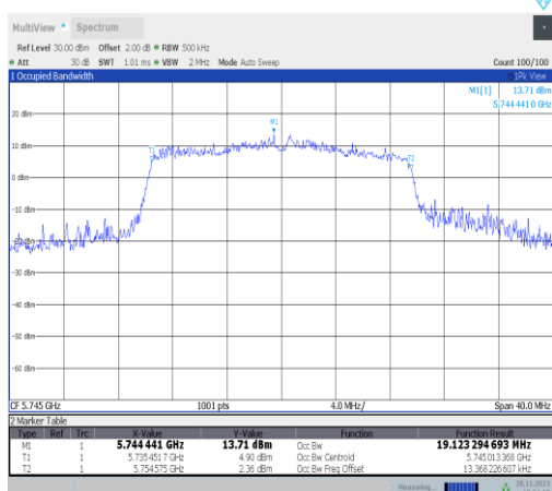
11ax20MIMO-Ant22-5745
