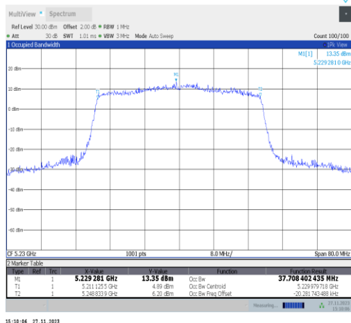
11ax40MIMO-Ant22-5230
