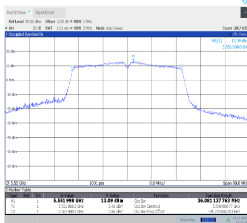
11n40MIMO-Ant25-5550
