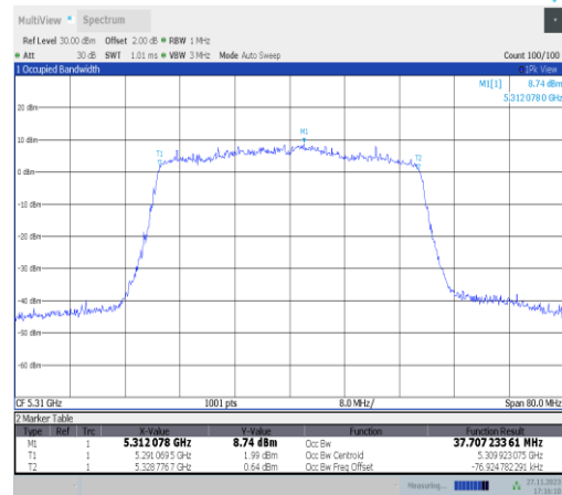
11ax40MIMO-Ant25-5310
