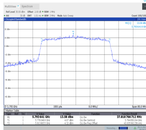
11ax40MIMO-Ant25-5795
