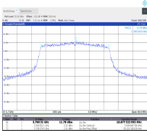
11ax20MIMO-Ant22-5700
