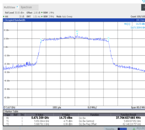
11ax40MIMO-Ant25-5670
