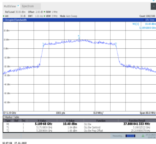
11ax40MIMO-Ant22-5190
