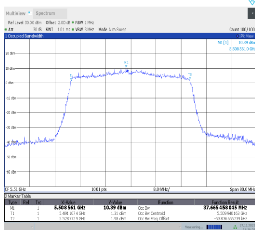
11ax40MIMO-Ant22-5510
