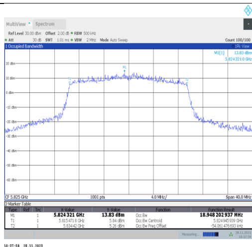
11ax20MIMO-Ant22-5825
