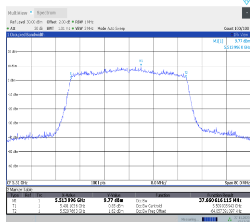
11ax40MIMO-Ant25-5510
