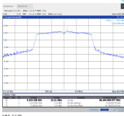
11n40MIMO-Ant25-5230
