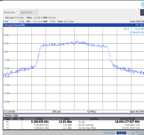
11ax20MIMO-Ant25-5260
