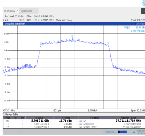
11ax40MIMO-Ant25-5710
