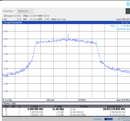
11ax20MIMO-Ant22-5500
