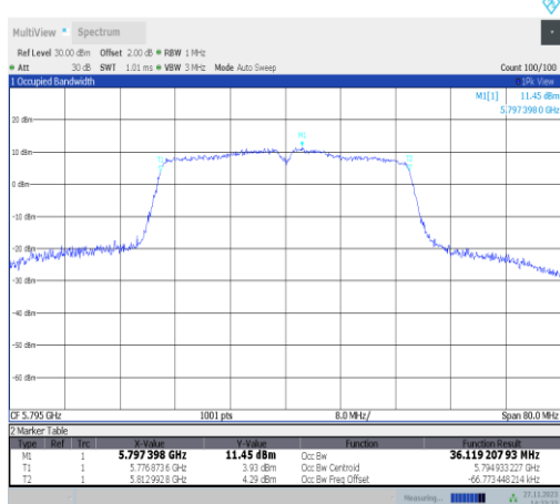
11n40MIMO-Ant22-5795
