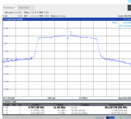
11n40MIMO-Ant25-5795
