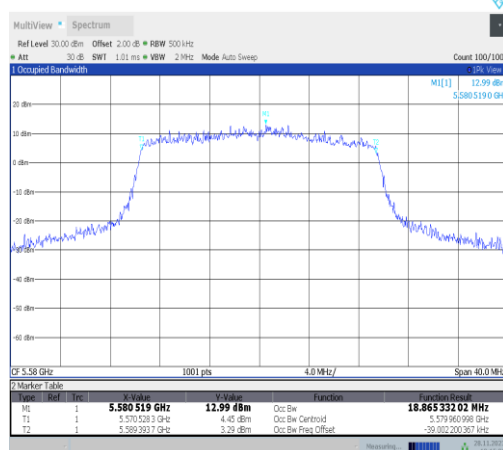
11ax20MIMO-Ant25-5580
