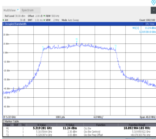
11ax20MIMO-Ant22-5320
