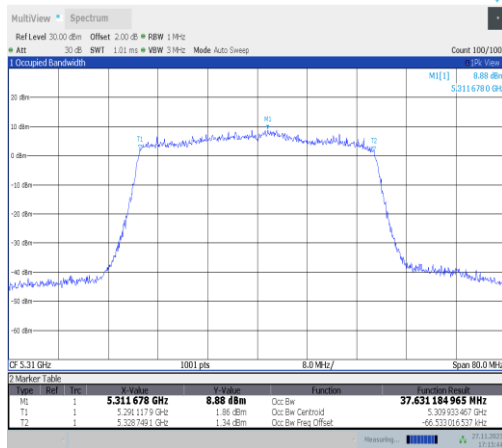
11ax40MIMO-Ant22-5310
