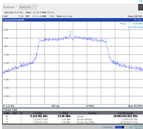
11ax20MIMO-Ant22-5220
