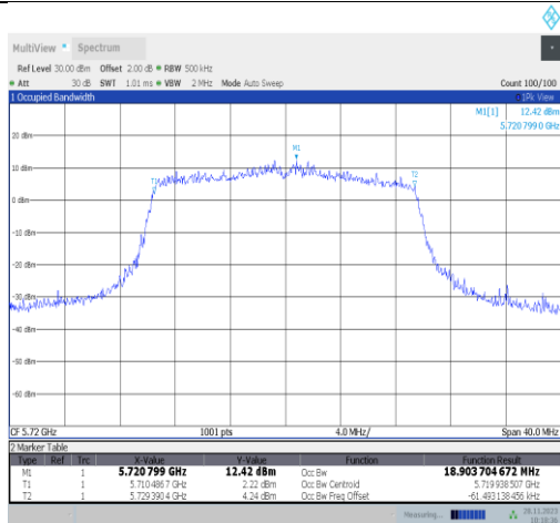
11ax20MIMO-Ant22-5720
