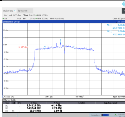
11ax40MIMO-Ant25-5755-PASS
