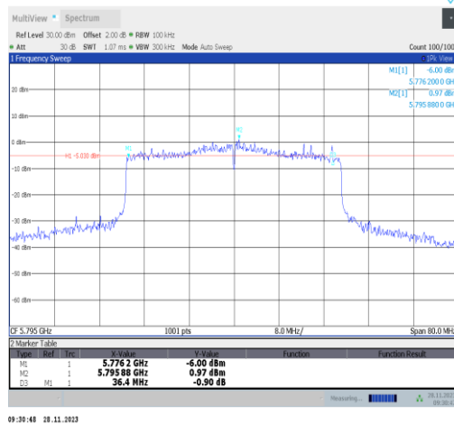
11ax40MIMO-Ant25-5795-PASS
