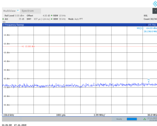
Band12-10MHz-QPSK-23060-1RB#0-Range2:0.15~30MHz
